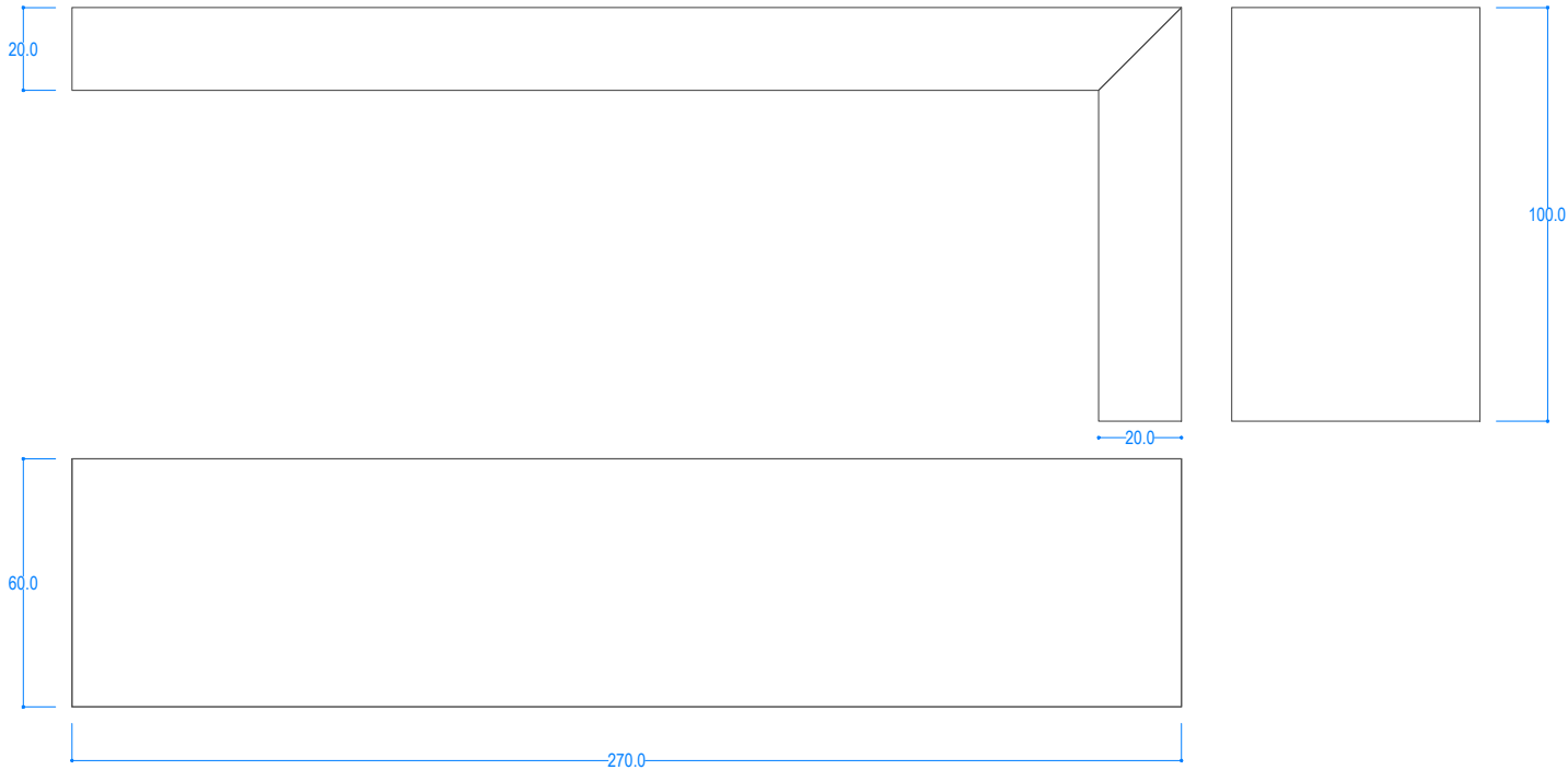
PEANYA 23 VISTA FRONTAL, LATERAL I PLANTA
