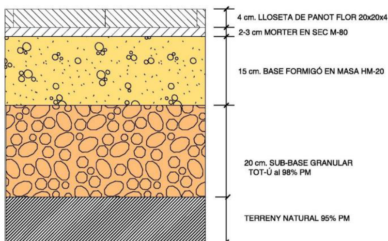
Detall 2. Capes ferm vorera.
