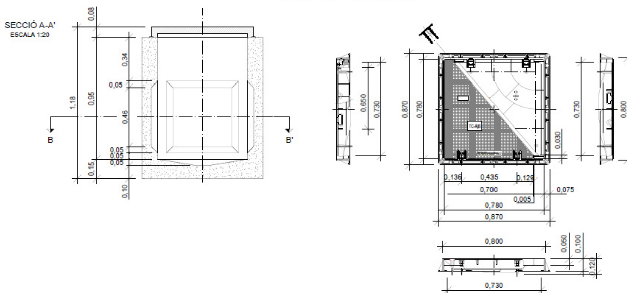
DETALL TAPA I MARC D'ARQUETA
