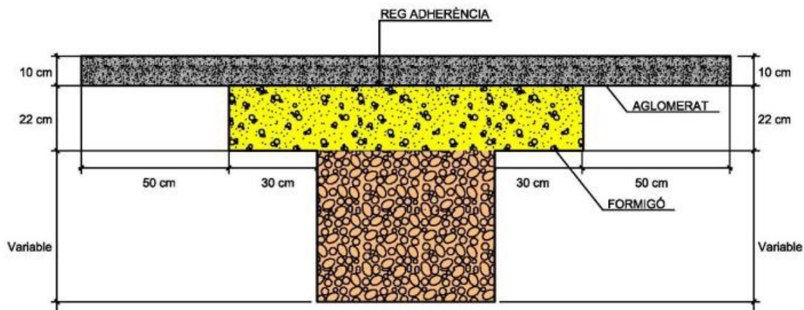
Detall 3. Zona de reposició. Sobreample calçada
