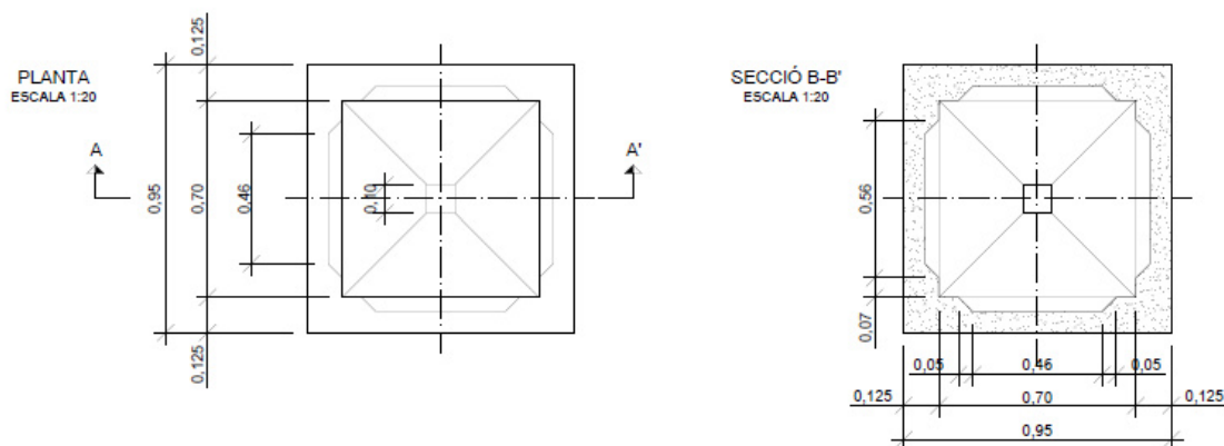
DETALL ARQUETA 2C 70x70cm Interior
