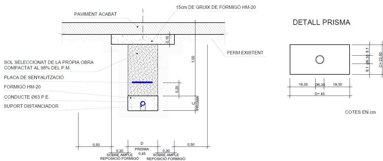
Detall 4. Detall tipus prisma formigó.
