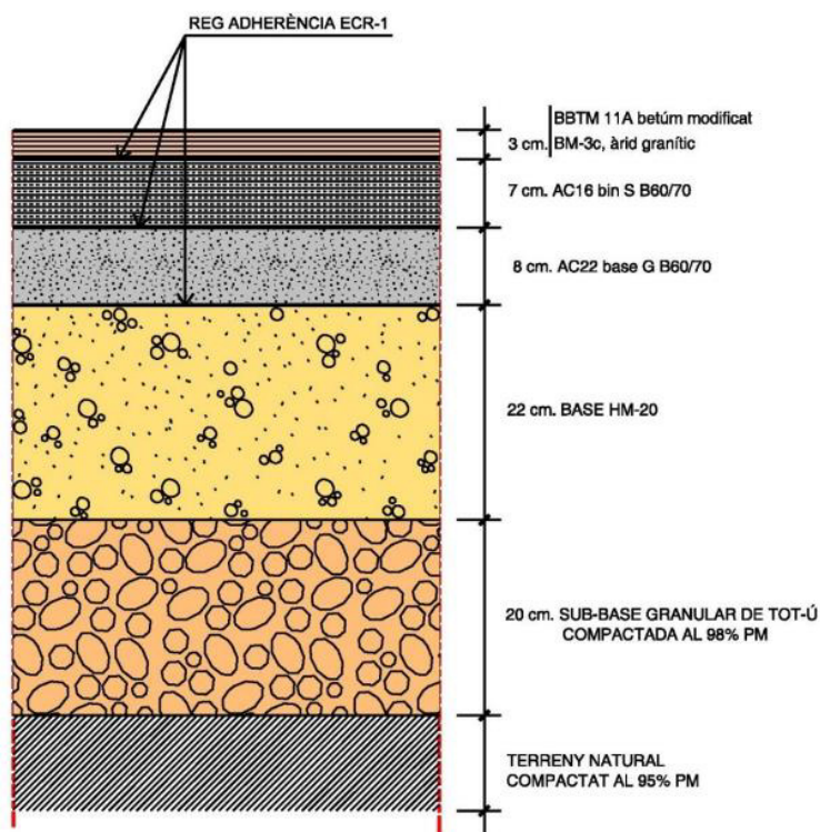
Detall 1. Capes ferm calçada. Xarxa bàsica
