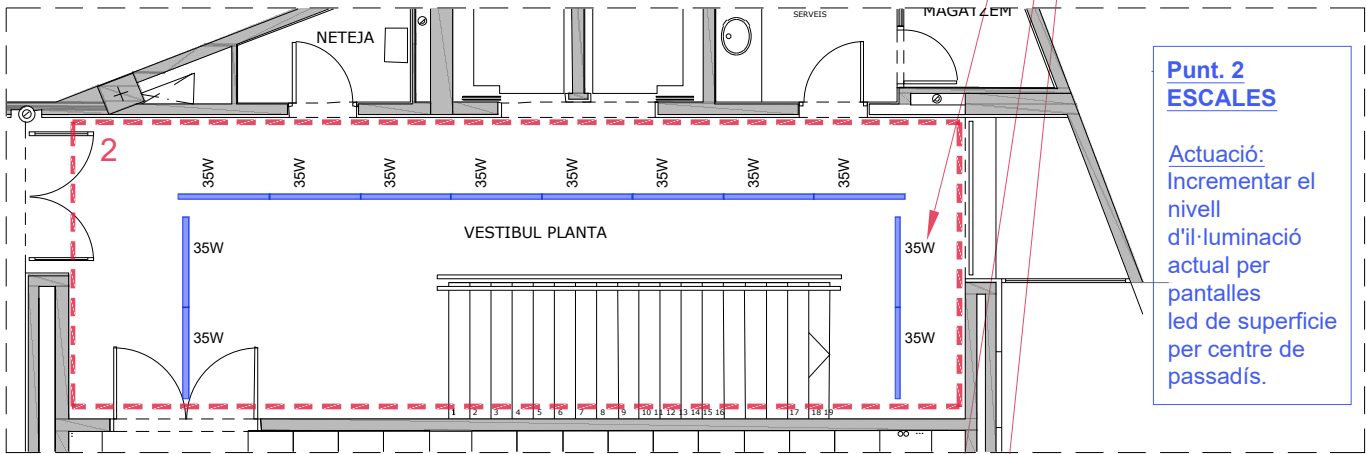
PLANTA 3
