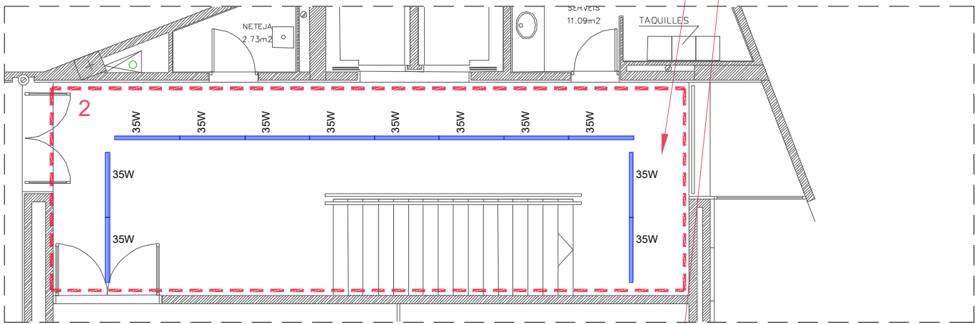
PLANTA 2
