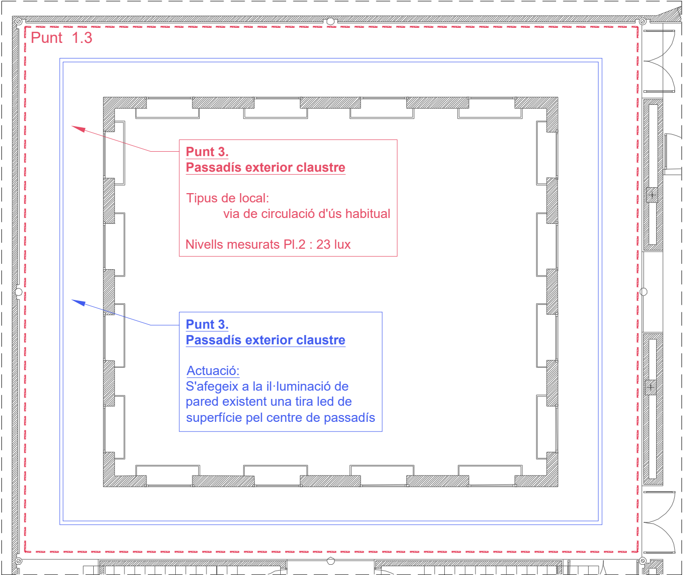
PLANTA 2
