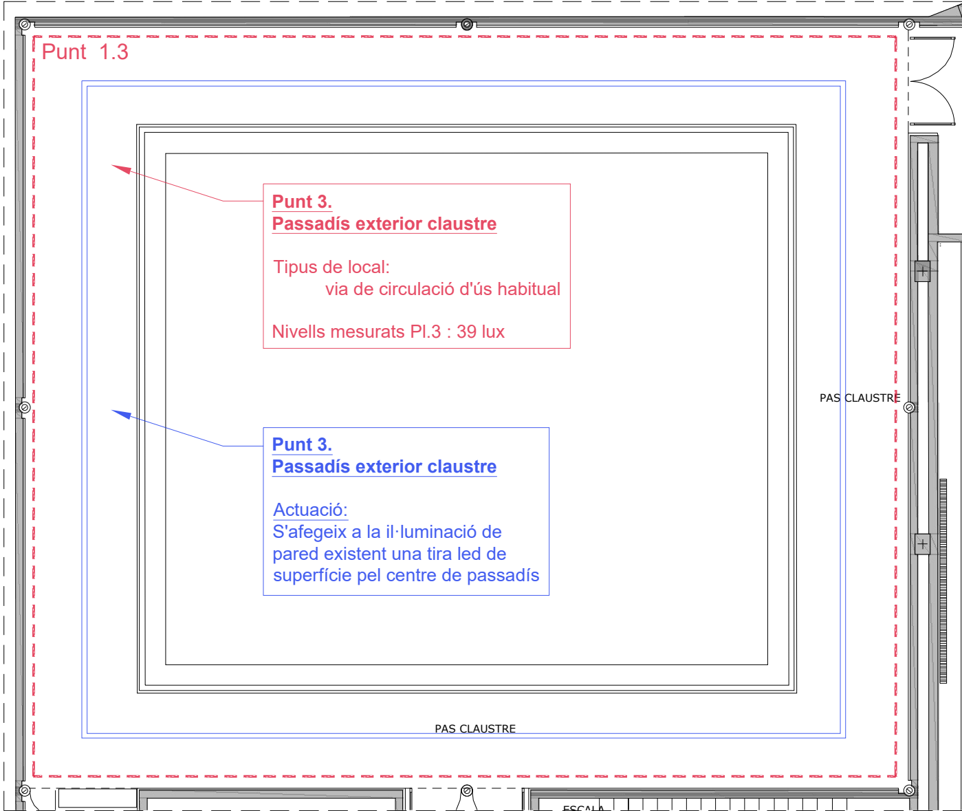
PLANTA 3
