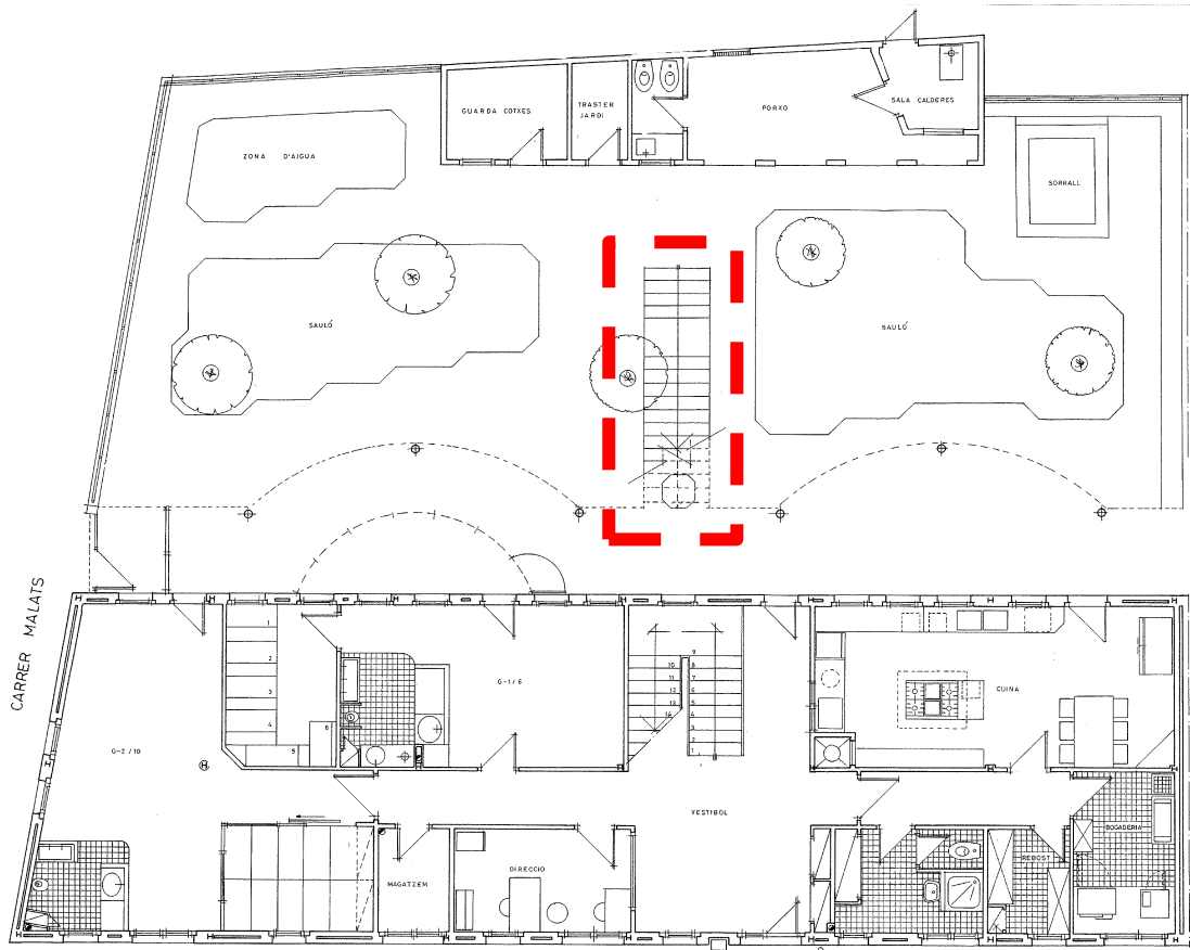
PLANTA BAIXA
