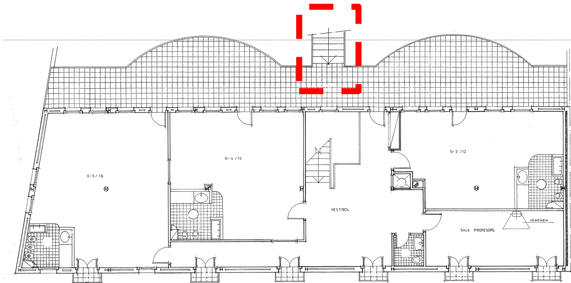
PLANTA BAIXA
