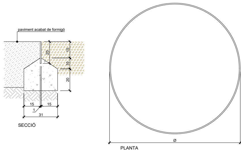
ESCOCELLS Ø120cm, Ø200cm, Ø250cm h=20cm e=1cm D'ACER GALVANITZAT Esc.: 1/10 (cotes en cm)
