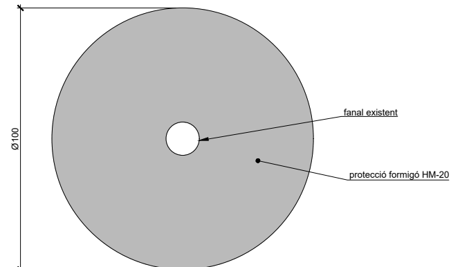
DETALL SUPORT DE FORMIGÓ HM-20 PER A FANAL EXISTENT A PARTERRE Esc.: 1/10 (cotes en cm)
