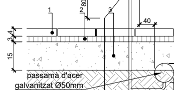
1 passamà d'acer galvanitzat Ø50mm 2 reg. d'adherència ECR-1 (1,0kg/m²) 3 base de formigó HM-20 e=15cm
