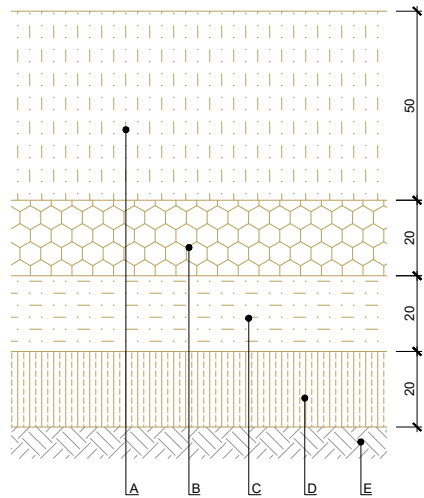
A terra vegetal adobada 50cm B terra sorrenca 20cm C ull de perdiu 20cm D gravetes filtrants 20cm E terreny natural fresat i airejat e=5cm
