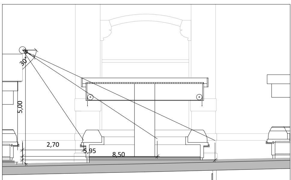
DETALL ACCÉS CARRER SANT MEDIR 1. Difusió realitzada amb toveres a 5.00 m alçada amb diferents cobertures
