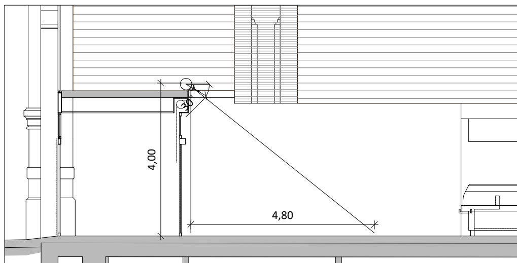
DETALL ACCÉS CARRER SANT MEDIR 2. Difusió realitzada amb toveres a 4.00 m alçada
