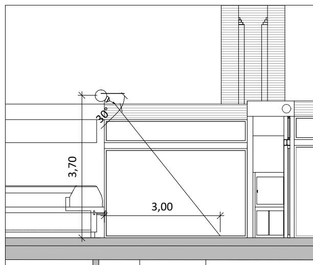
DETALL ACCÉS SUPERMERCAT2. Difusió realitzada amb toveres
