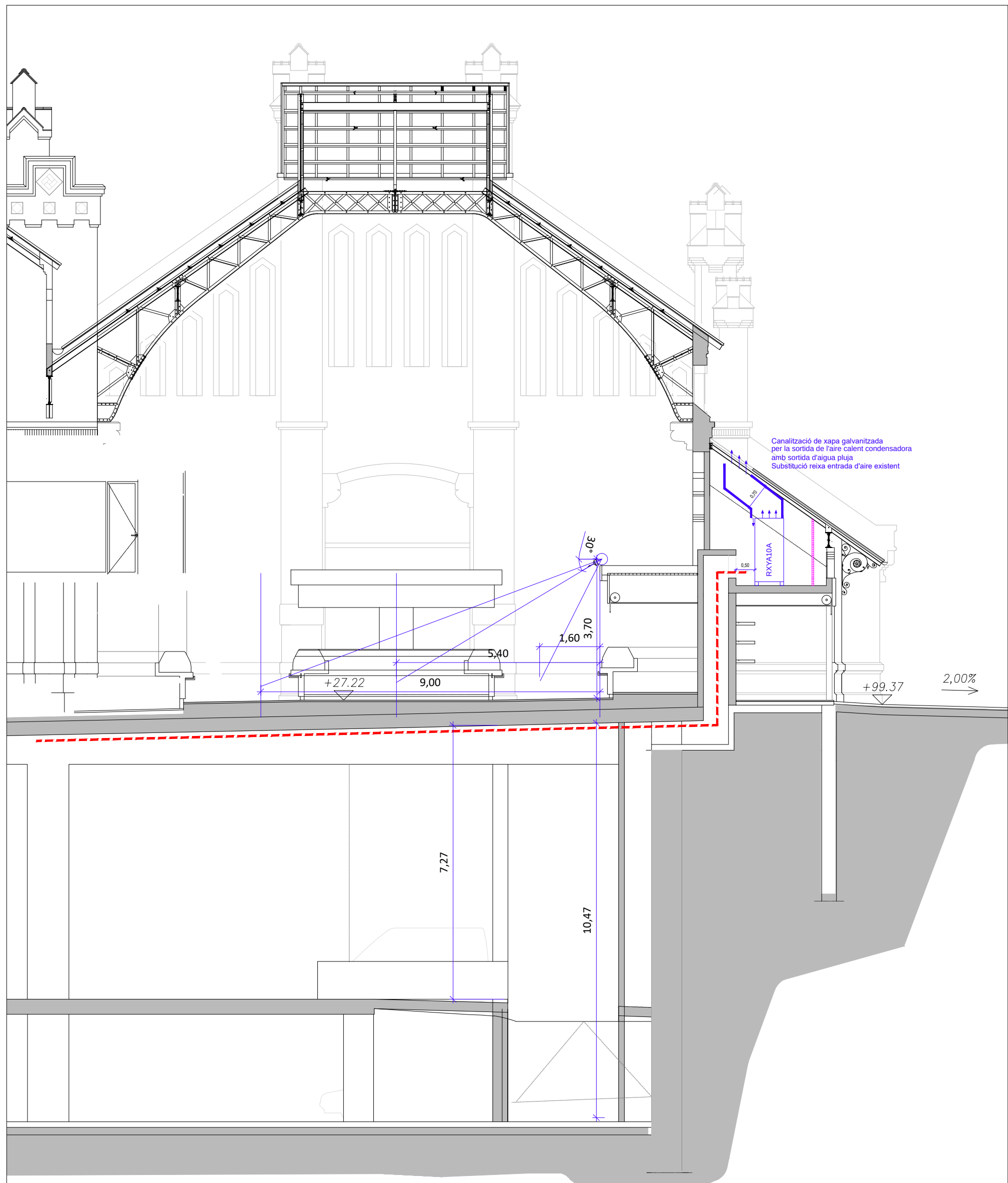
DETALL PUJADA CABLEJAT A SALA DE MÀQUINES I PARADES PERIMETRAIS CARRER CACERES
