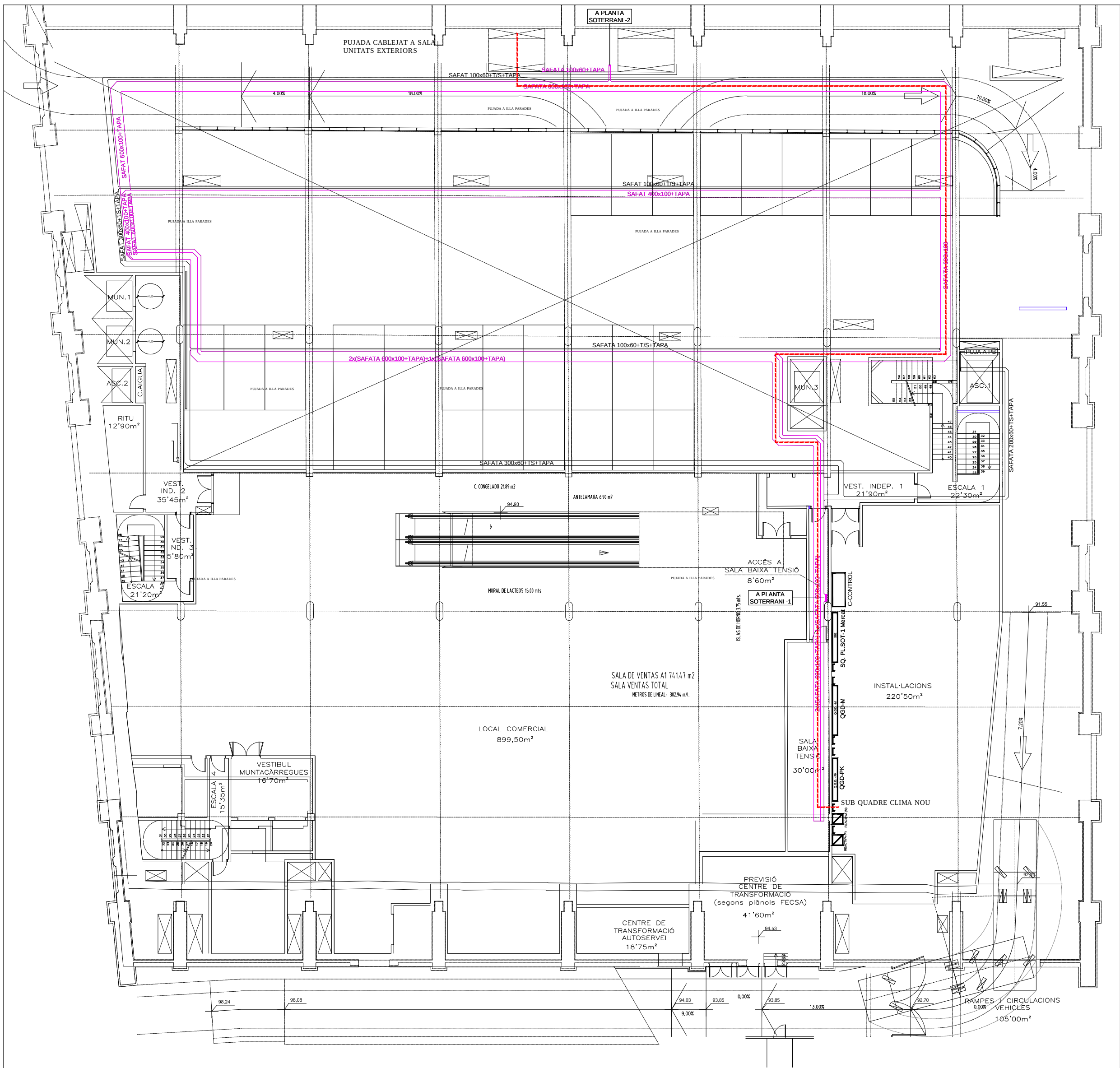
DETALL QUADRE ELÈCTRIC PRINCIPAL I DISTRIBUCIÓ DE SAFATES EXISTENTS EN PLANTA SOTERRANI -1
