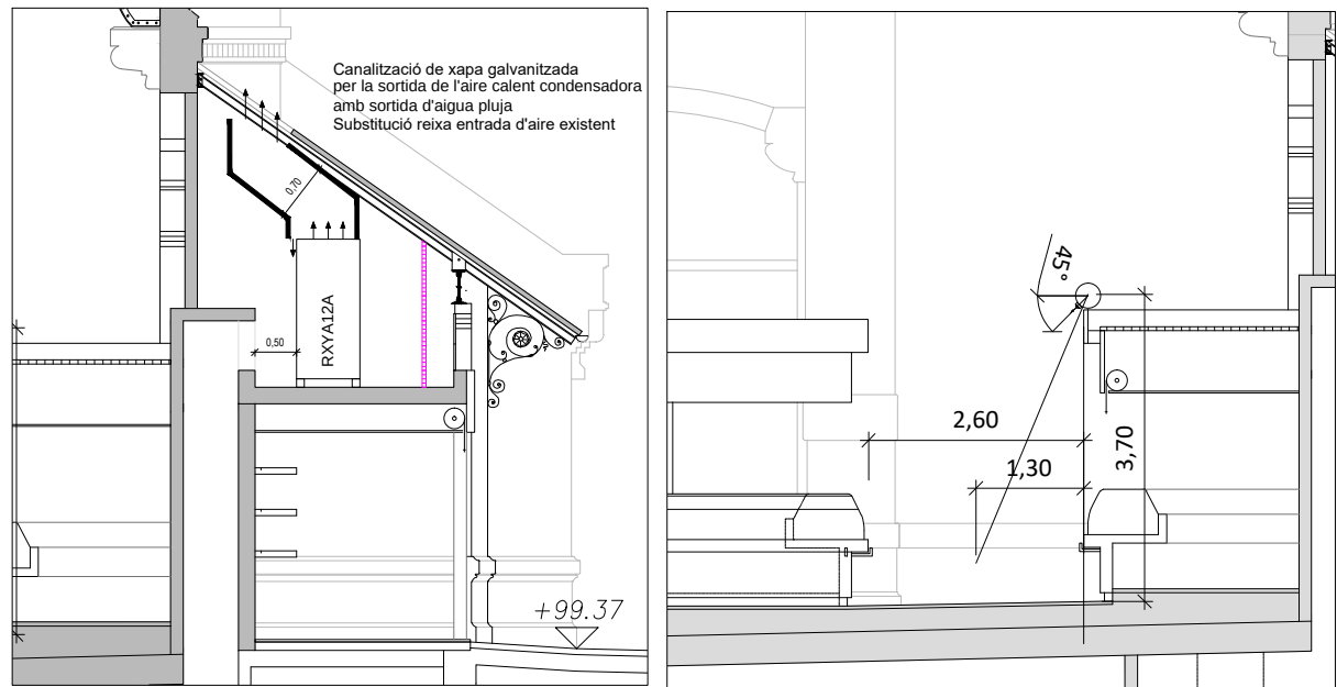
DETALL PASSADIS I ACCÉS CÀCERES: Difusió realitzada amb Multi toveres a 3.70 m alçada a centre de passadís
