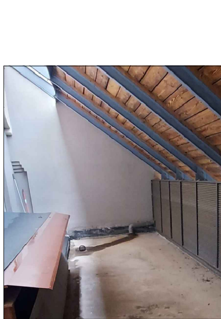
DETALL SALES DE MÀQUINES: Unitats exteriors en terrassa exterior serà necessari substituir reixa lateral aportació d'aire
