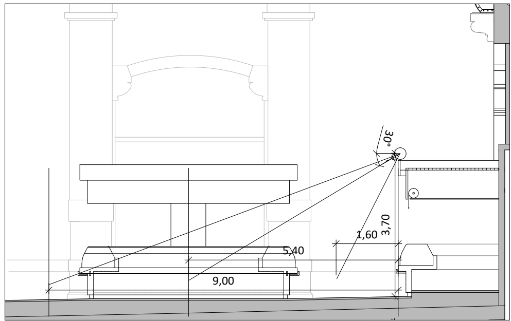
DETALL ACCÉS CARRER SANT JORDI. Difusió realitzada amb toveres a 3.70 m alçada amb diferents cobertures
