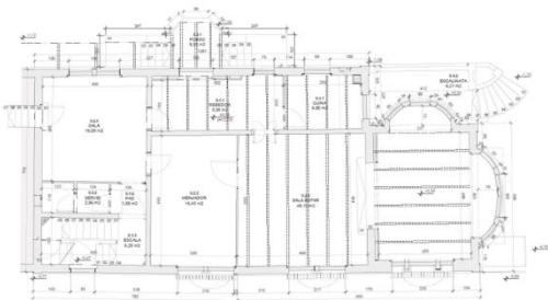
PLANTA BAIXA
