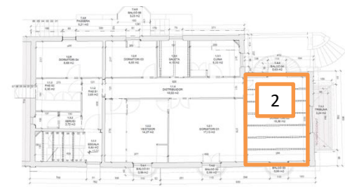
PLANTA PIS
