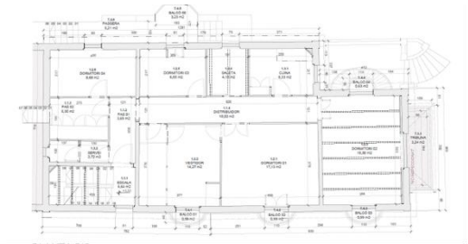
PLANTA PIS
