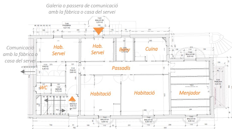
PLANTA PIS
