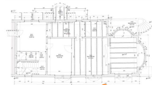
PLANTA BAIXA
