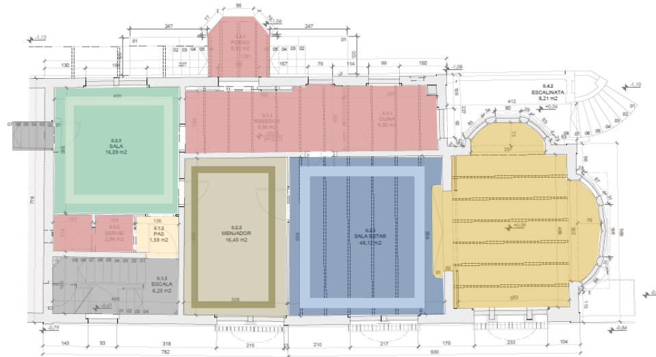
PLANTA BAIXA
