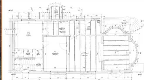
PLANTA BAIXA
