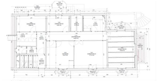
PLANTA PIS
