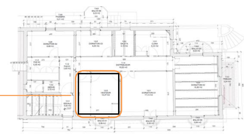
PLANTA PIS
