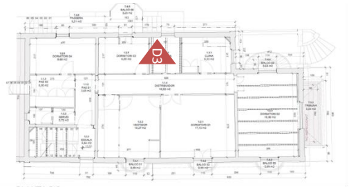
PLANTA PIS
