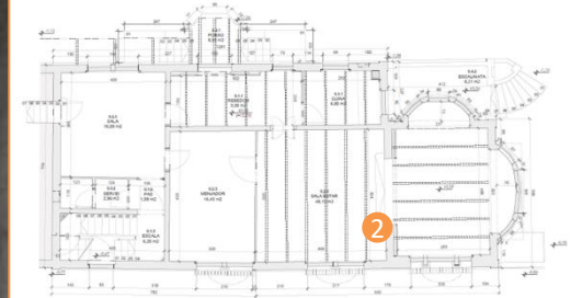
PLANTA BAIXA
