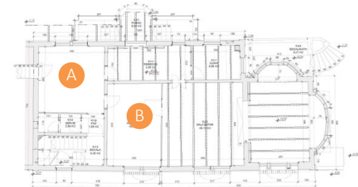
PLANTA BAIXA
