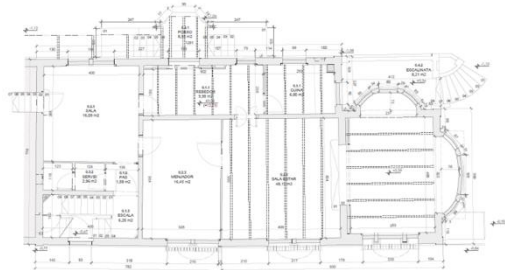
PLANTA BAIXA
