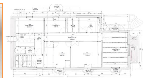
PLANTA PIS
