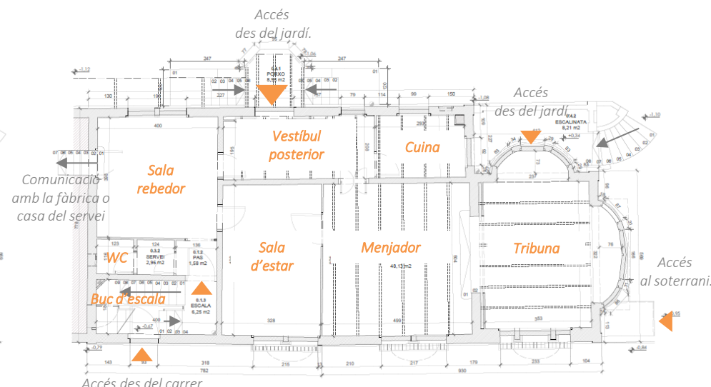
PLANTA BAIXA
