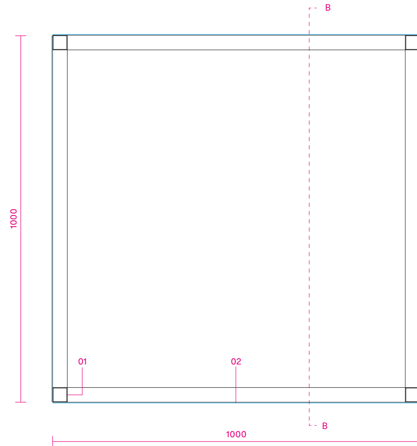
SECCIÓ HORITZONTAL A - ESC. 1:10
