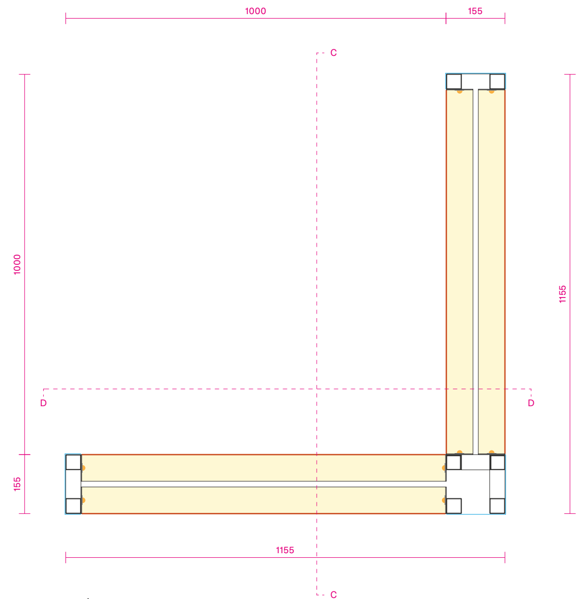
SECCIÓ HORITZONTAL B - ESC. 1:10
