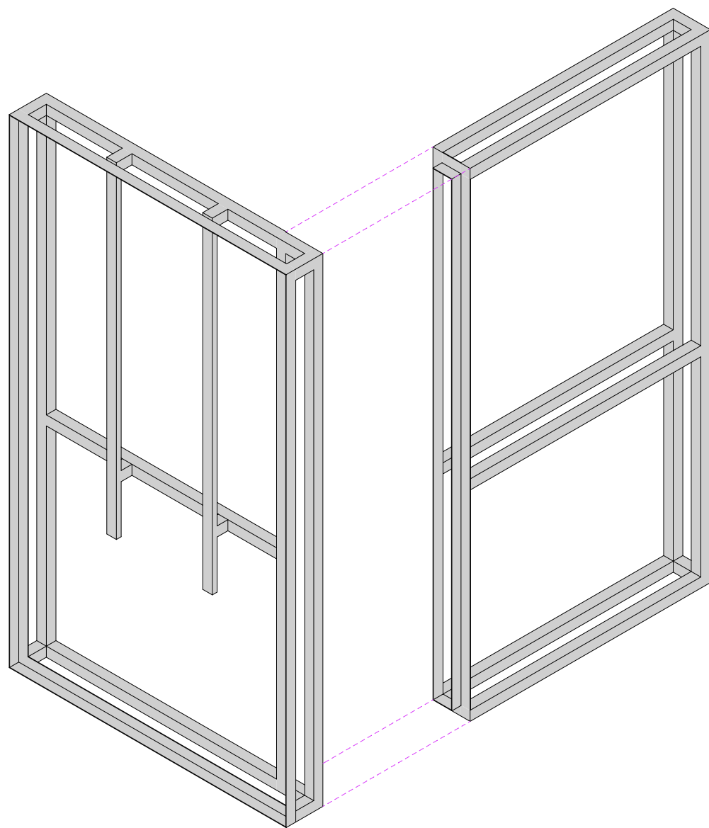
01 / FIXACIÓ DE LES DUES ESTRUCTURES
