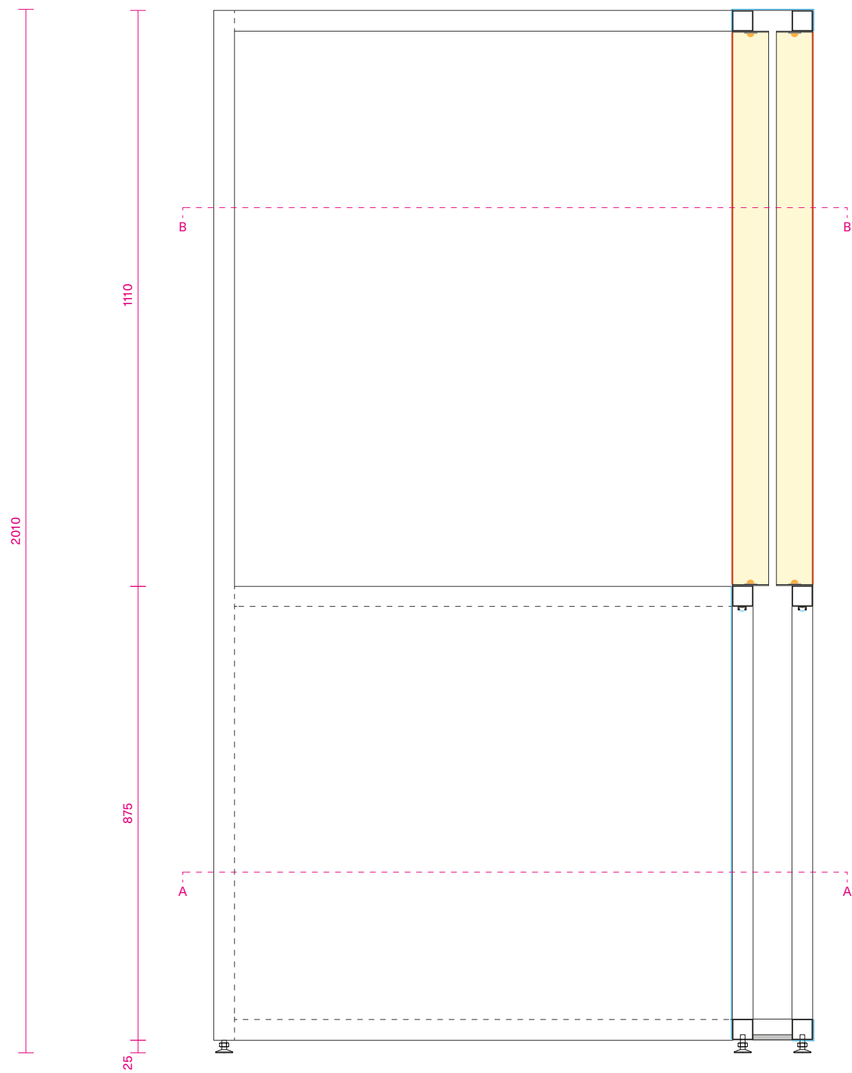
SECCIÓ VERTICAL C - ESC. 1:10
