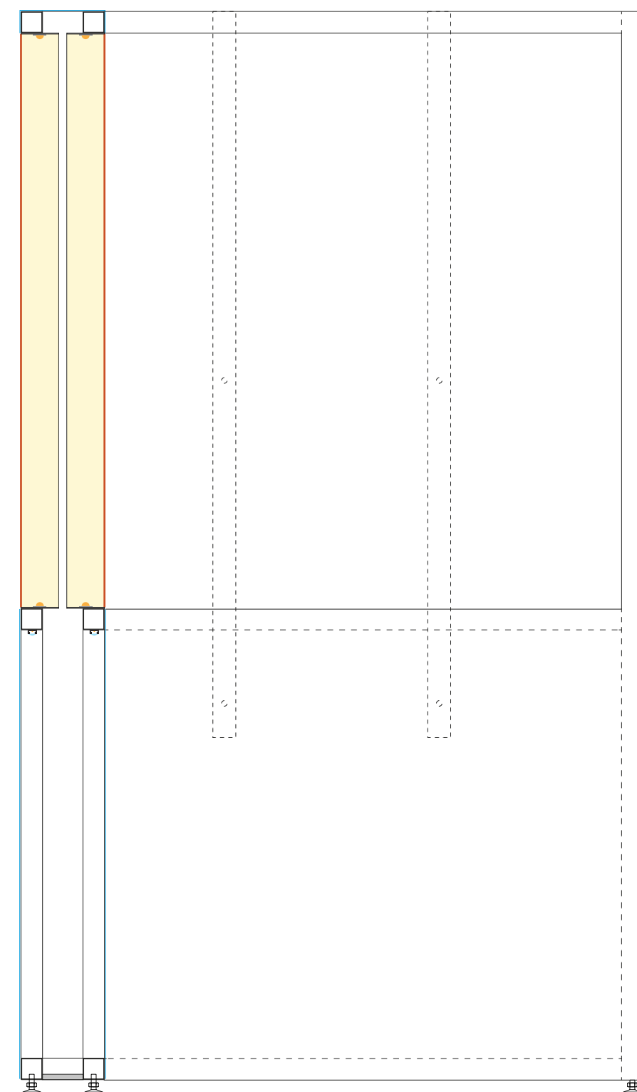
SECCIÓ VERTICAL D - ESC. 1:10
