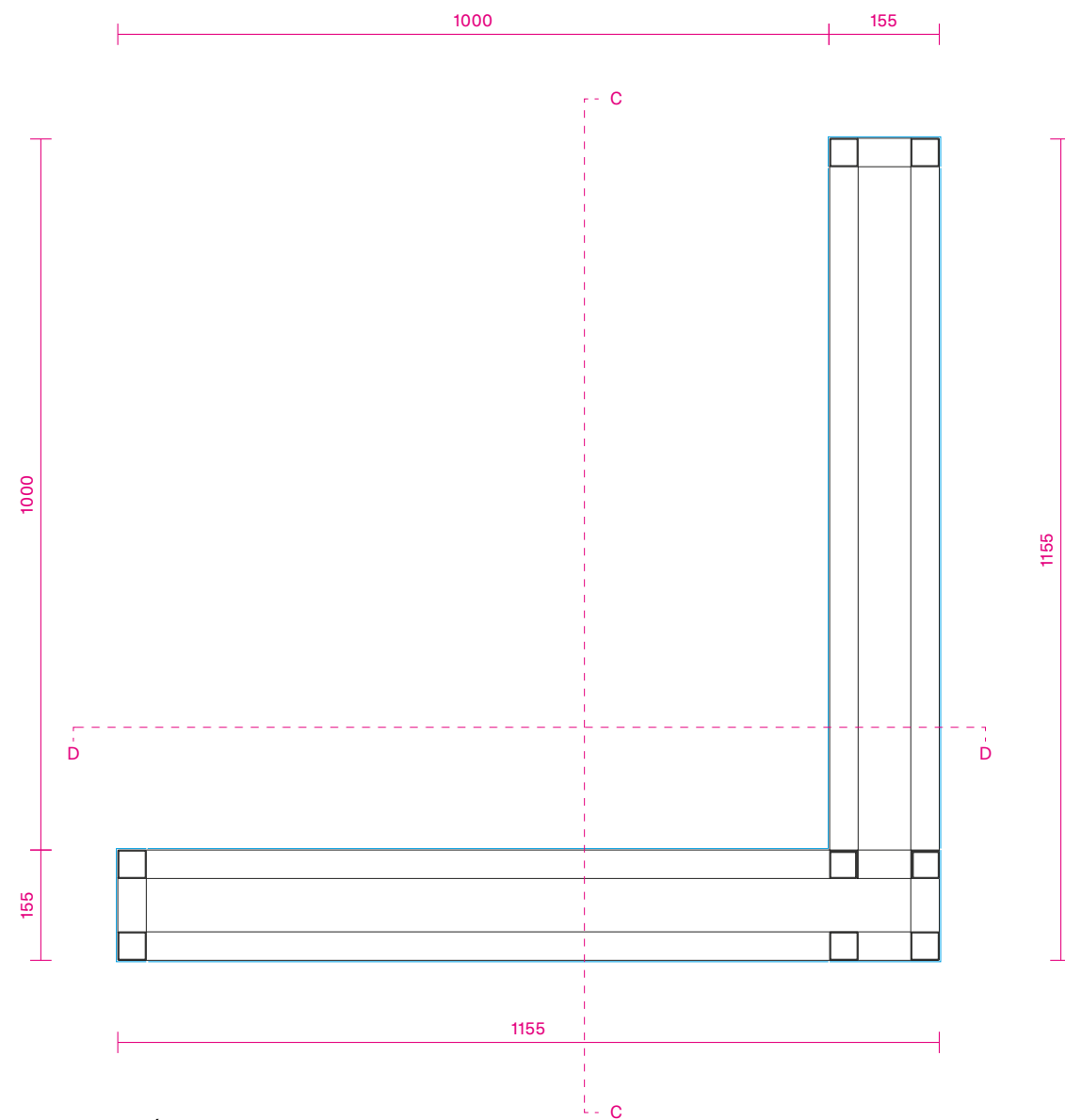
SECCIÓ HORITZONTAL A - ESC. 1:10
