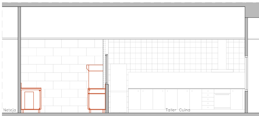
SECCIÓ 3
