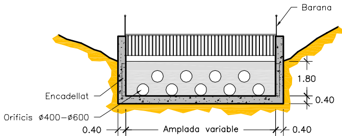
SECCIÓ B-B'
