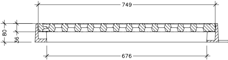
SECCIÓ
