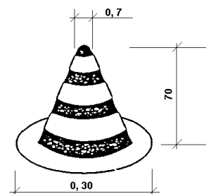
CONO BALIZAMIENTO
