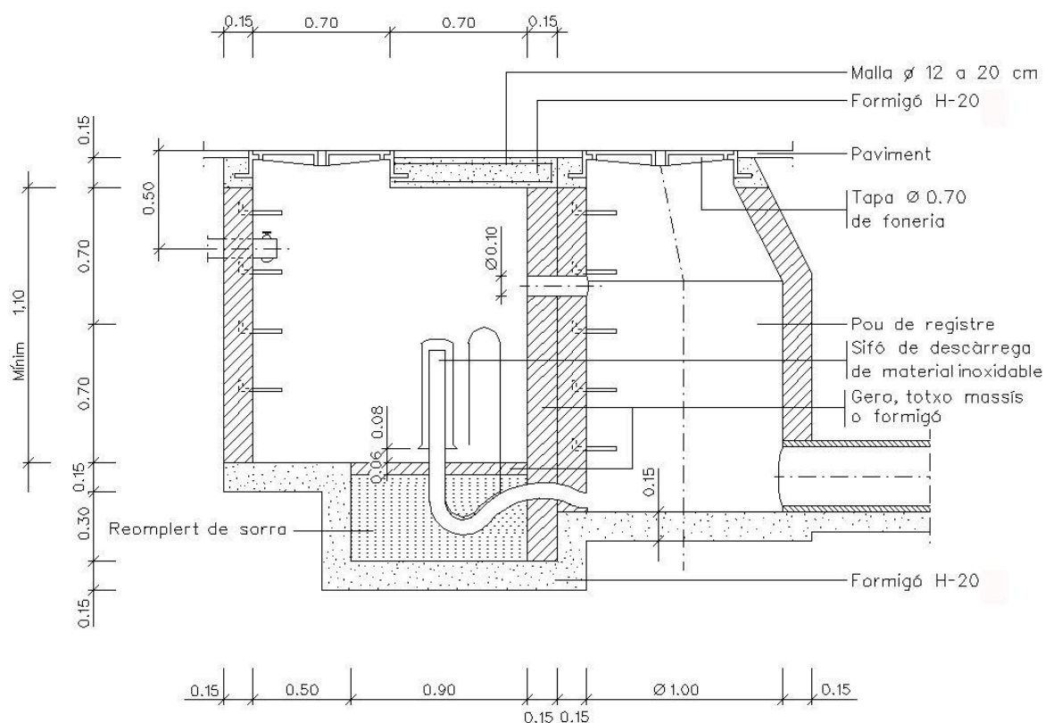
Càmbra de decàrrega amb pou
