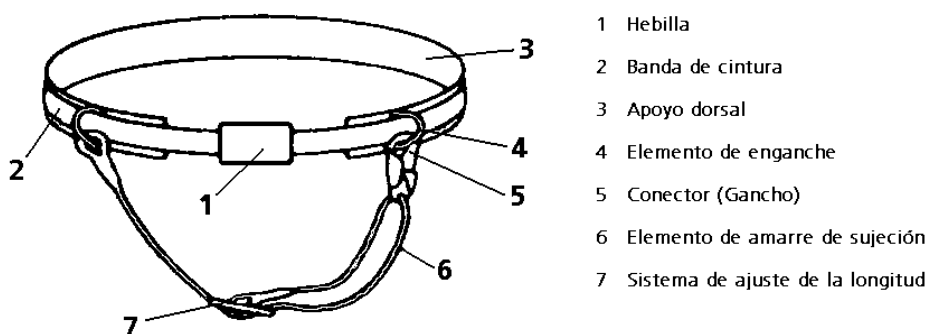
Cinturón de sujeción con elemento de amarre incorporado
