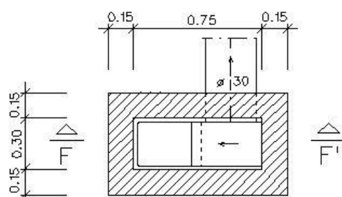
SECCI6 F-F'
