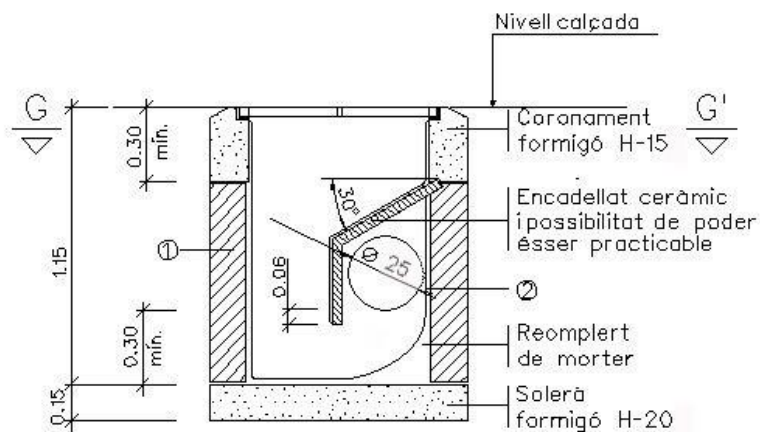
SECCI6 F-F'
