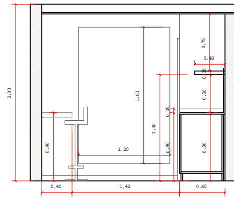
SECCIÓ 2 PROPUESTA
