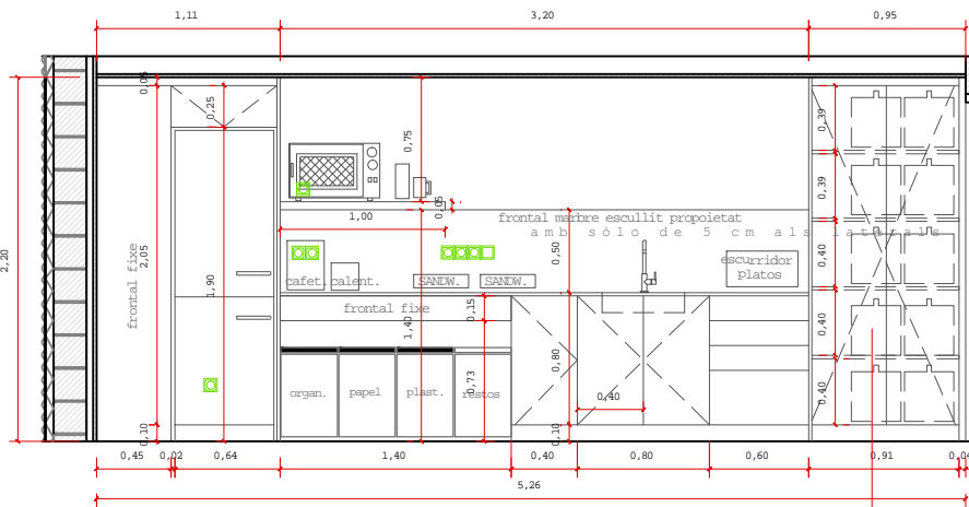
SECCIÓ 3 PROPUESTA
