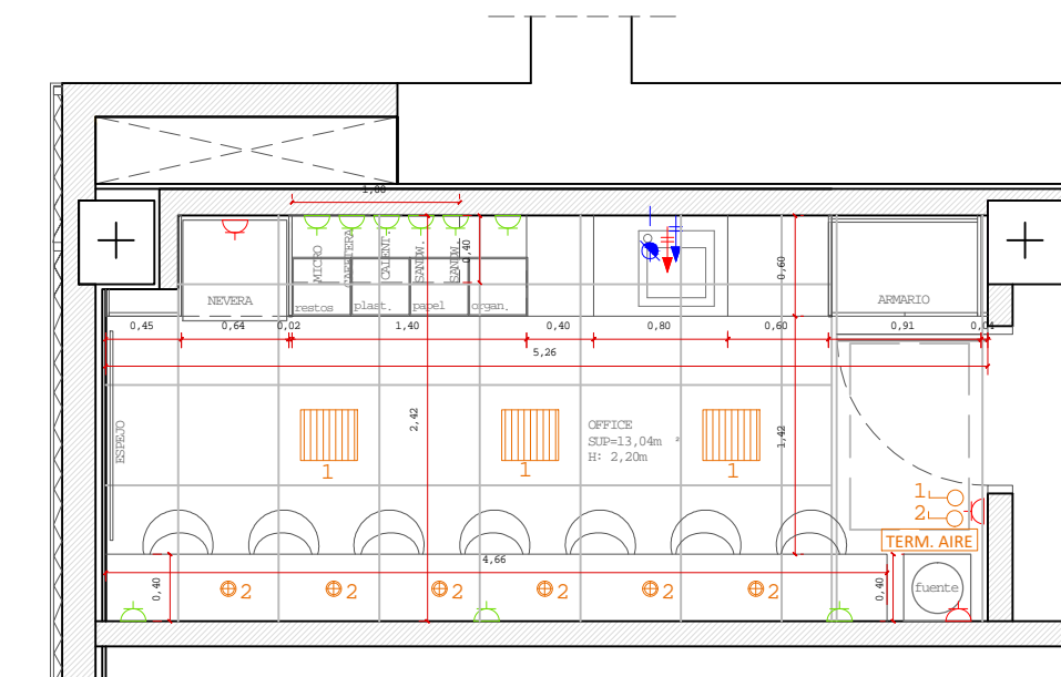
PLANTA PROPUESTA
