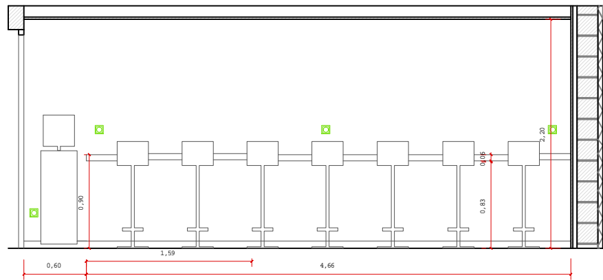
SECCIÓ 1 PROPUESTA
