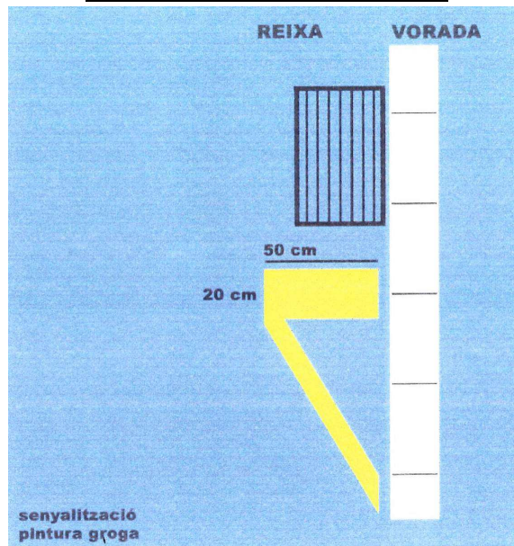
FIGURA 2 EJEMPLO SEÑALIZACION REJA
