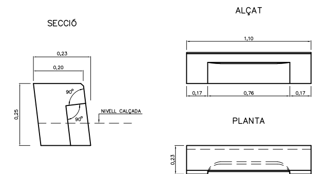
VORADA GRANÍTICA BÚSTIA
