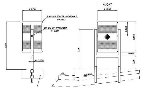
PAPERERA BARCELONA 70L ESCALA 1:20
