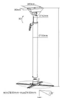
PRB-16-01L
