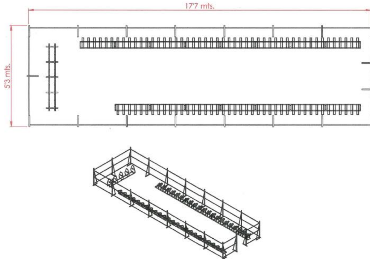
Proposta de disseny dels recintes d'aparcaments de bicicletes i VMP
