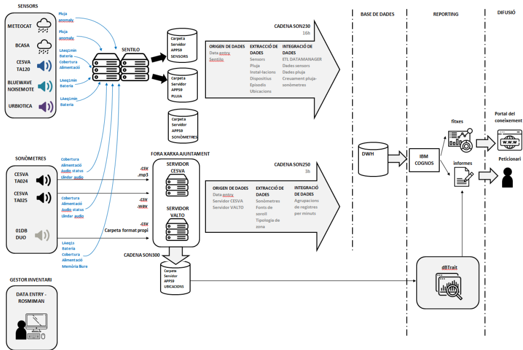
Fig 1. Estructura de gestió de la xarxa de monitorització del soroll
