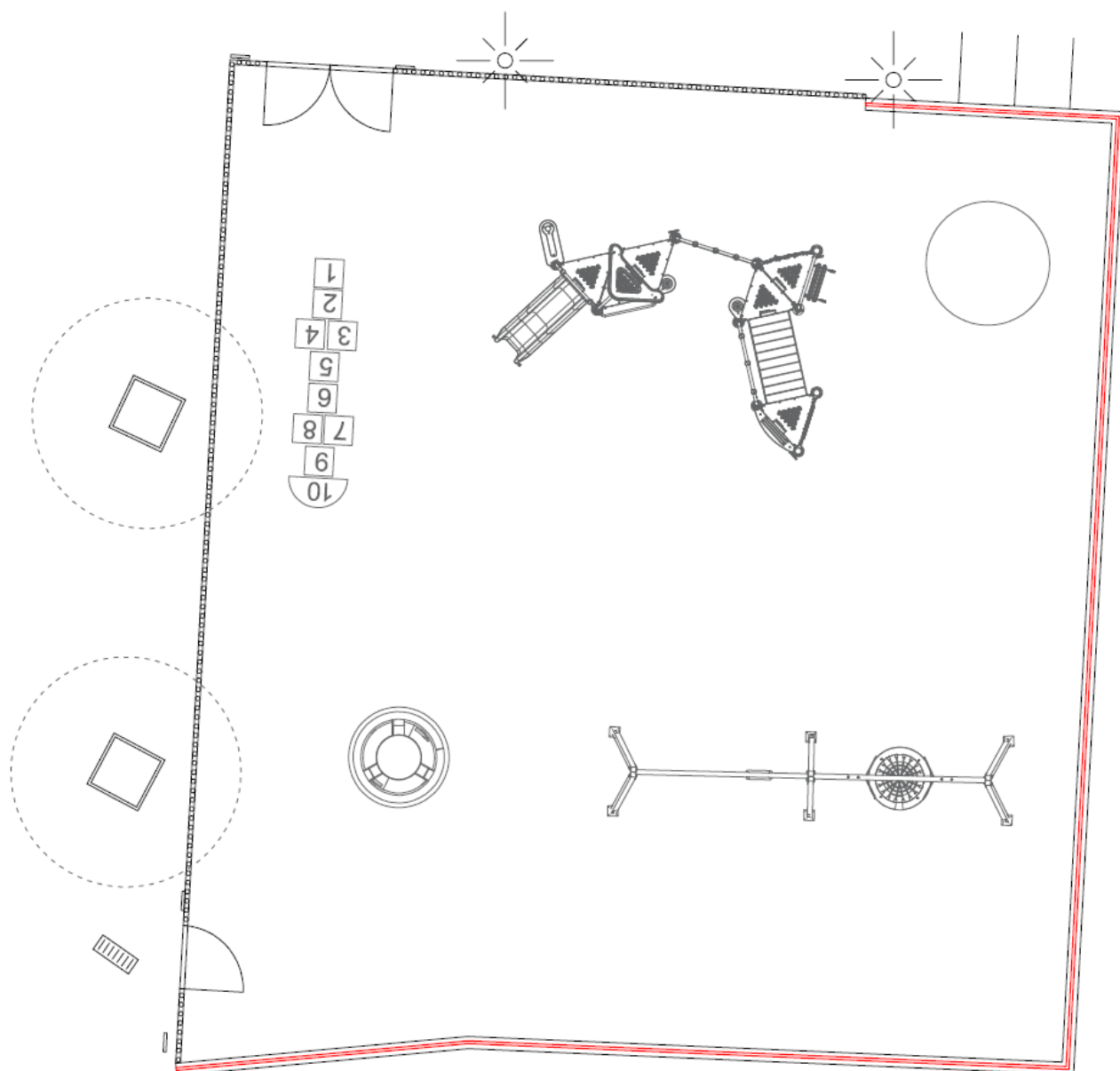
Planta de l'àrea de joc infantil i, indicat en color vermell, de la barana a instal·lar.
