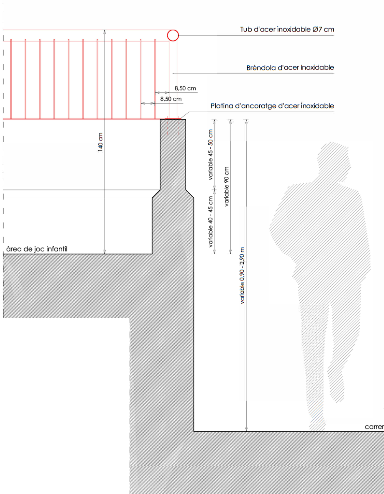
Secció tipus i alçat de la barana a instal·lar.
