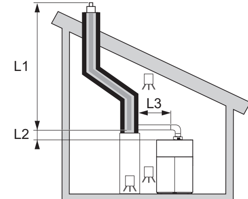
Fig.71 Conductos de humos flexibles B 23p
