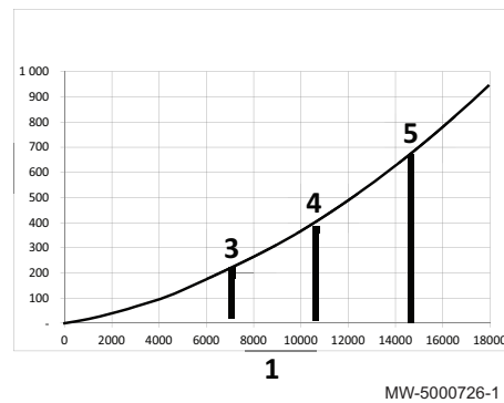
Fig.20 Caídas de presión para POWER HT Plus 250
