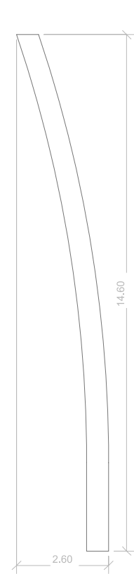
Secció diapasó
