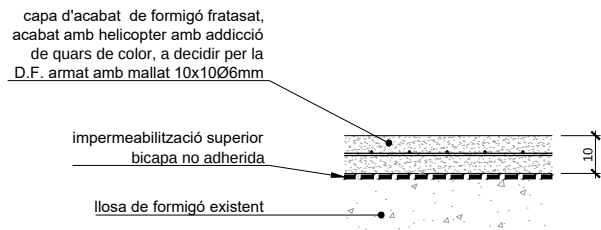
REPOSICIÓ DE PAVIMENT DE FORMIGÓ esc.: 1/10 (cotes en cm)
