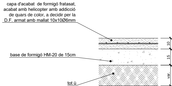
PAVIMENT DE FORMIGÓ (nou paviment) esc.: 1/10 (cotes en cm)
