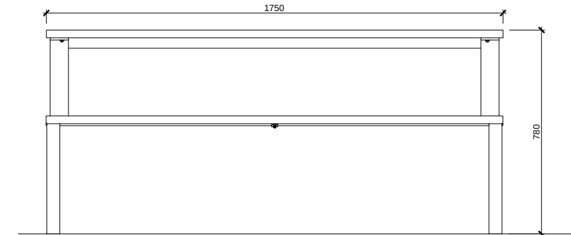
ALÇAT FRONTAL
