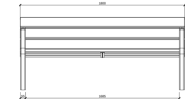
ALÇAT FRONTAL
