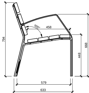
ALÇAT LATERAL
