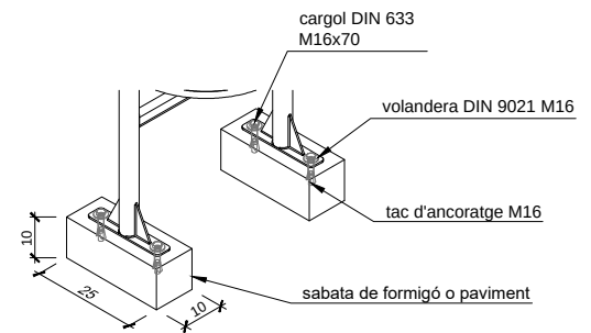
DETALL ANCRATGE A PAVIMENTS DURS
