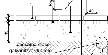
DETALL PAVIMENT DE MICROAGLOMERAT Esc.: 1/10 (cotes en cm)
