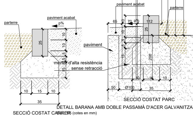
VORADA TIPUS Tauló de 100x25x15cm Esc.: 1/10 (cotes en cm)
