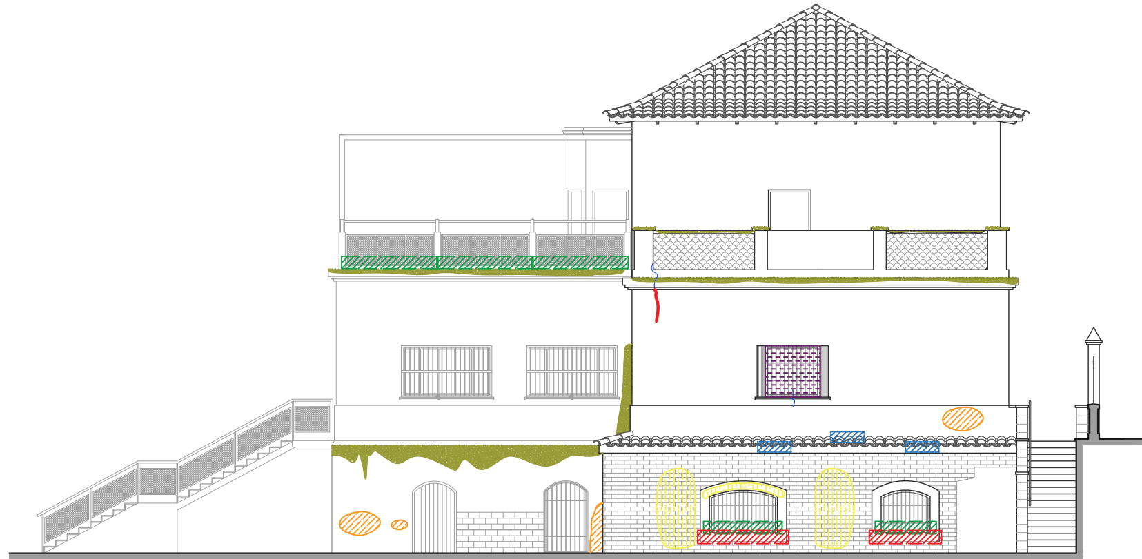
FAÇANA LATERAL (C/PADILLA)
