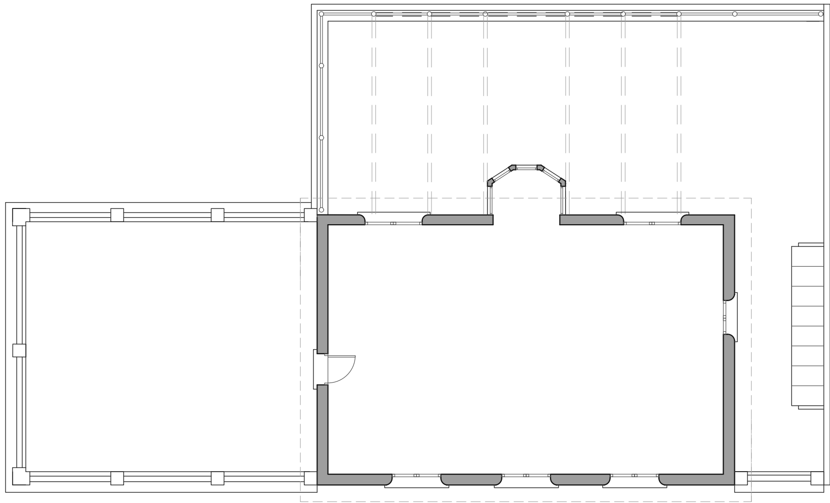
PLANTA PRIMERA
