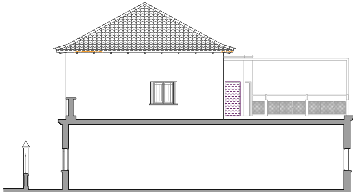
FAÇANA LATERAL (C/MARINA)
