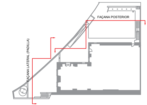
PLANTA SOTERRANI I JARDI
