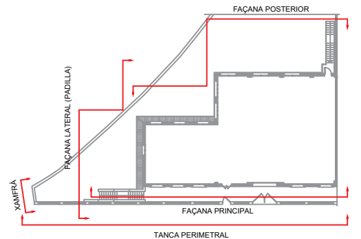
PLANTA BAIXA
