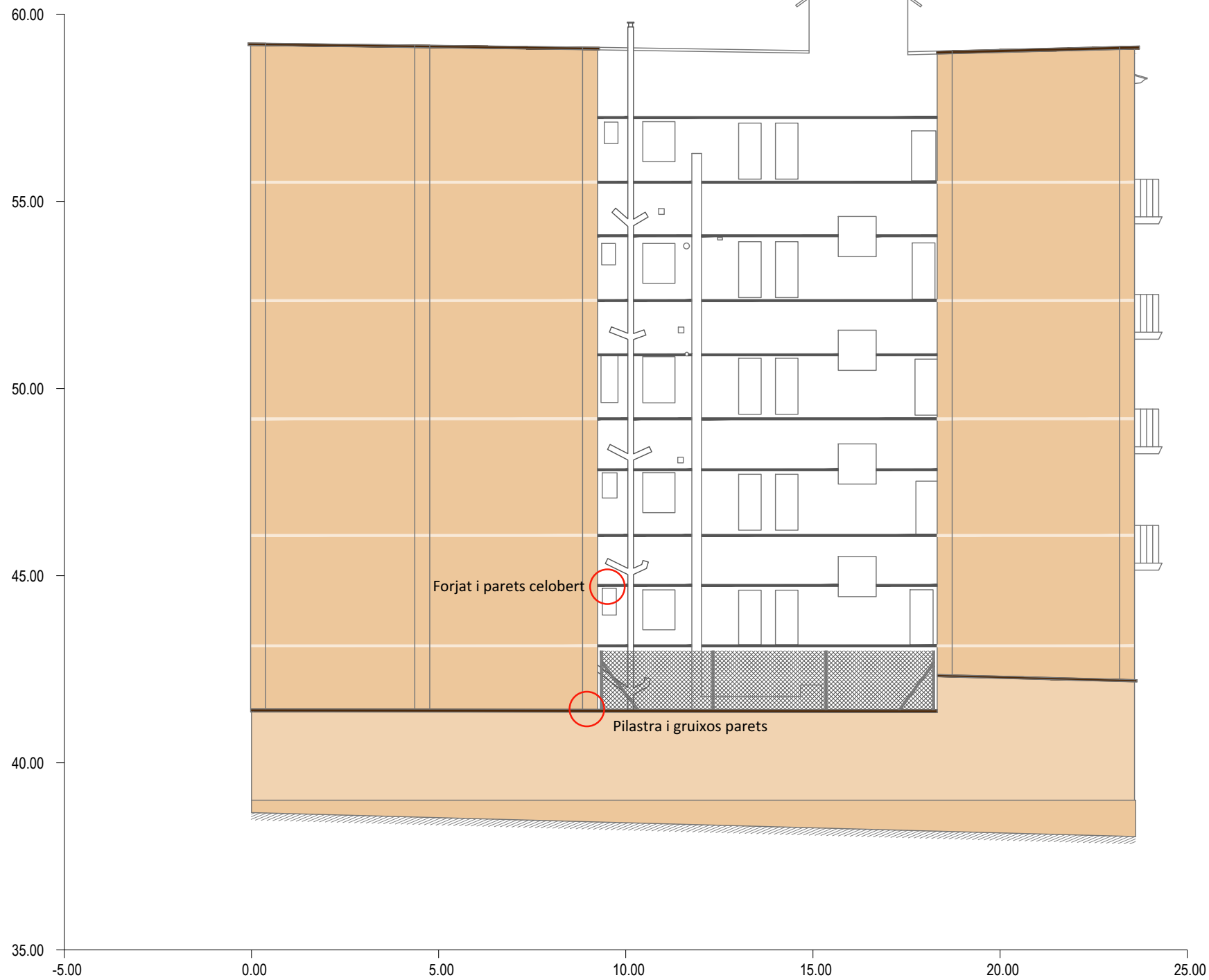
ALÇAT A1 Escala 1:150
