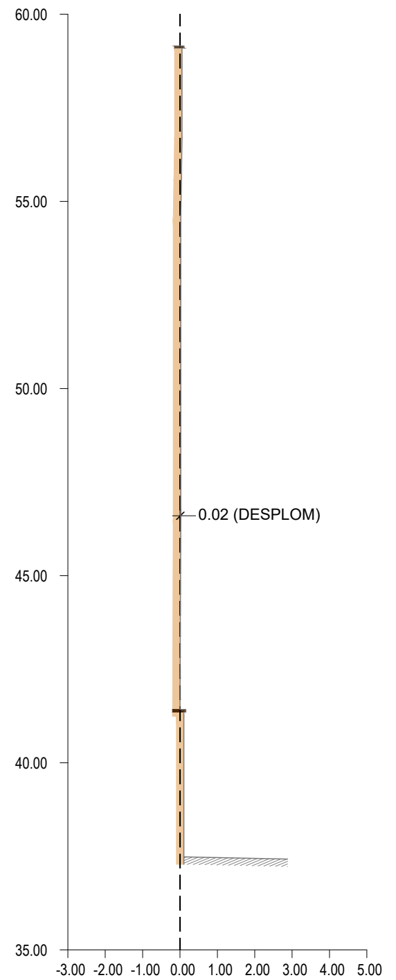
SECCIÓ S1 Escala 1:150
