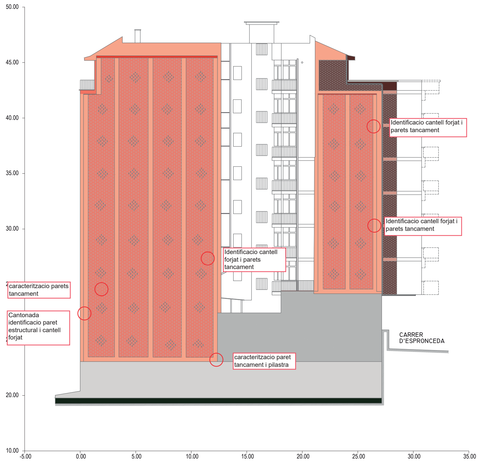
ALÇAT A1 Escala 1:200
