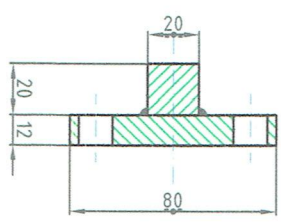
SECCION A-A
