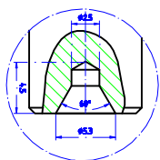
PUNTO CENTRALE A 2.5 DIN 332
