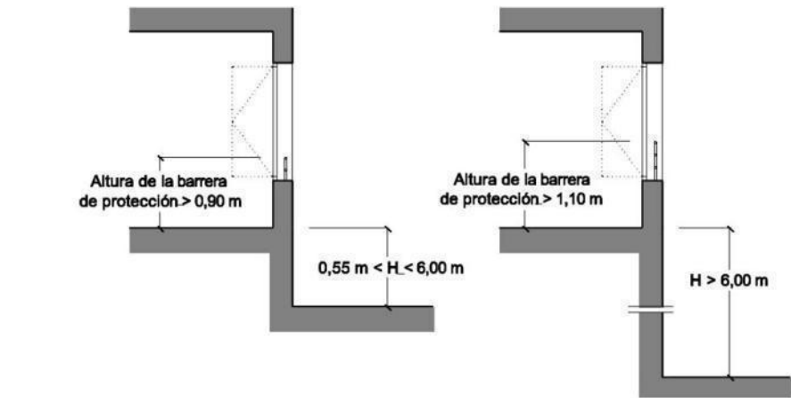
3) Figura 3.1 Barreras de protección en ventanas
