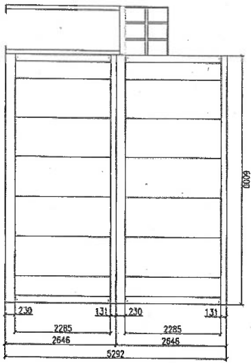
ALZADO POSTERIOR
