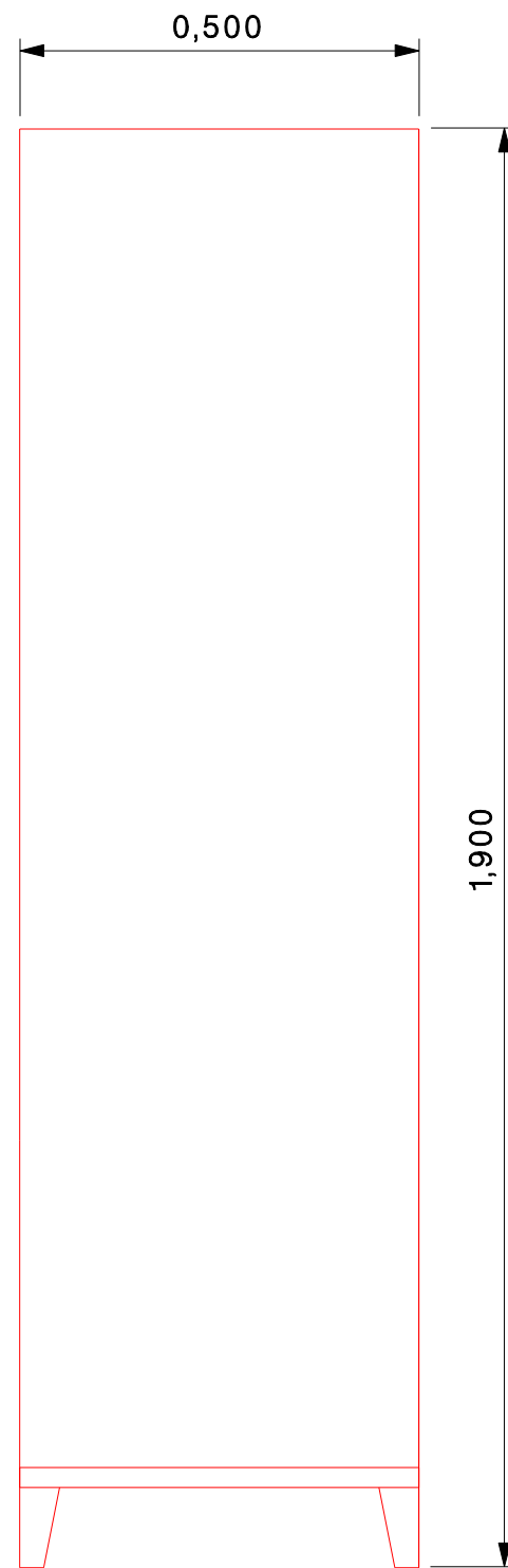
ALÇAT LATERAL EXTERIOR
