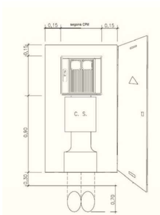
Esquema 1 enviat per Endesa de com s'ha d'instal·lar l'armari.
