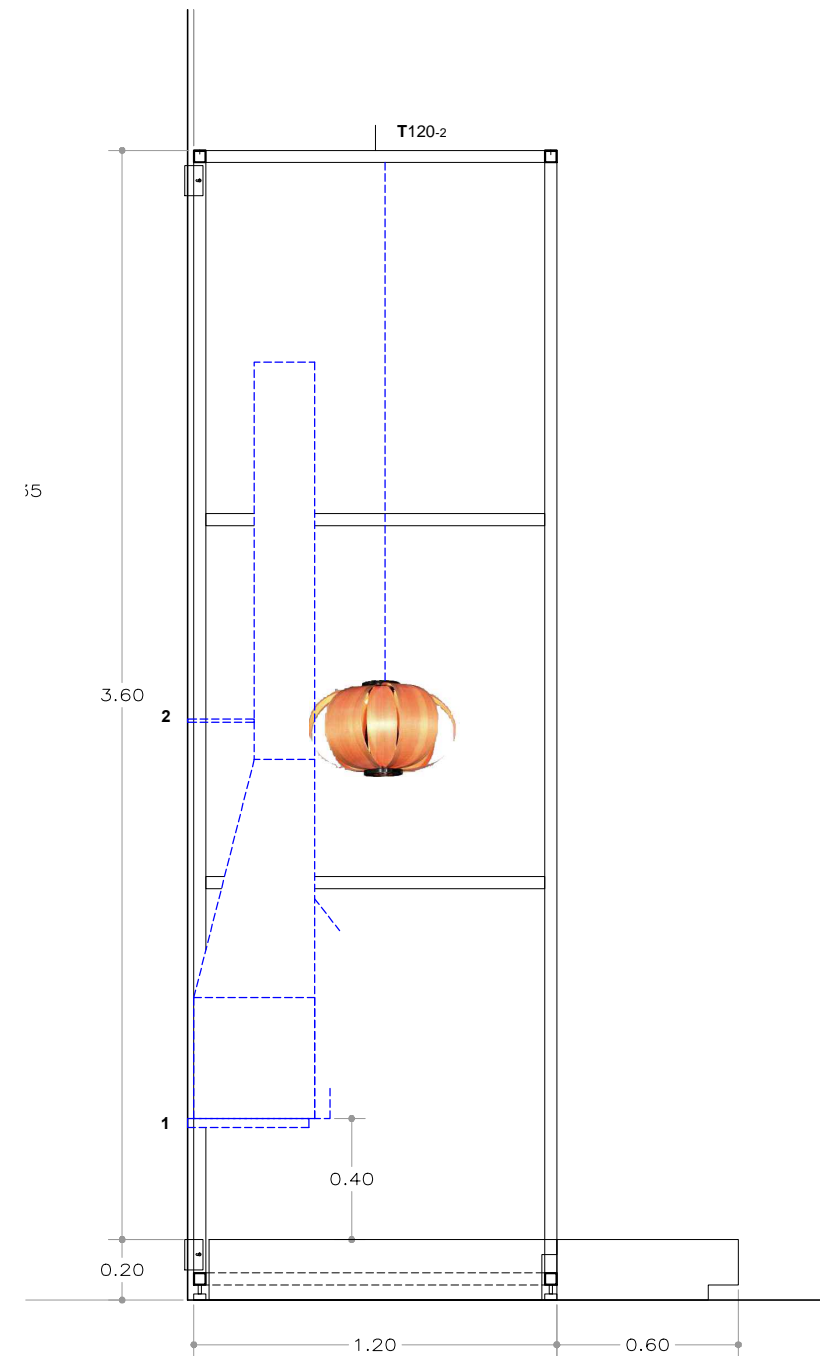
XEMENEIA CAPILLA FIJACIÓN A PARED (existente) 1 Marco inferior atornillado a pared 2 Varilla entre tiro y pared
