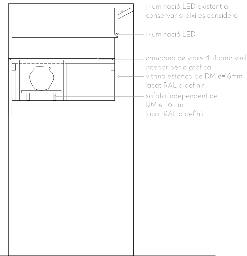
secció 1:10
