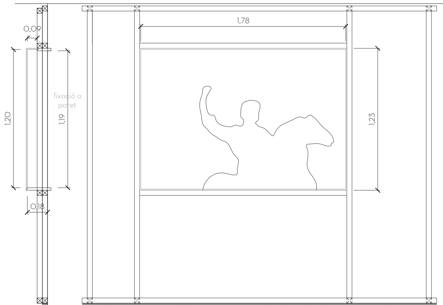
secció 1:20
