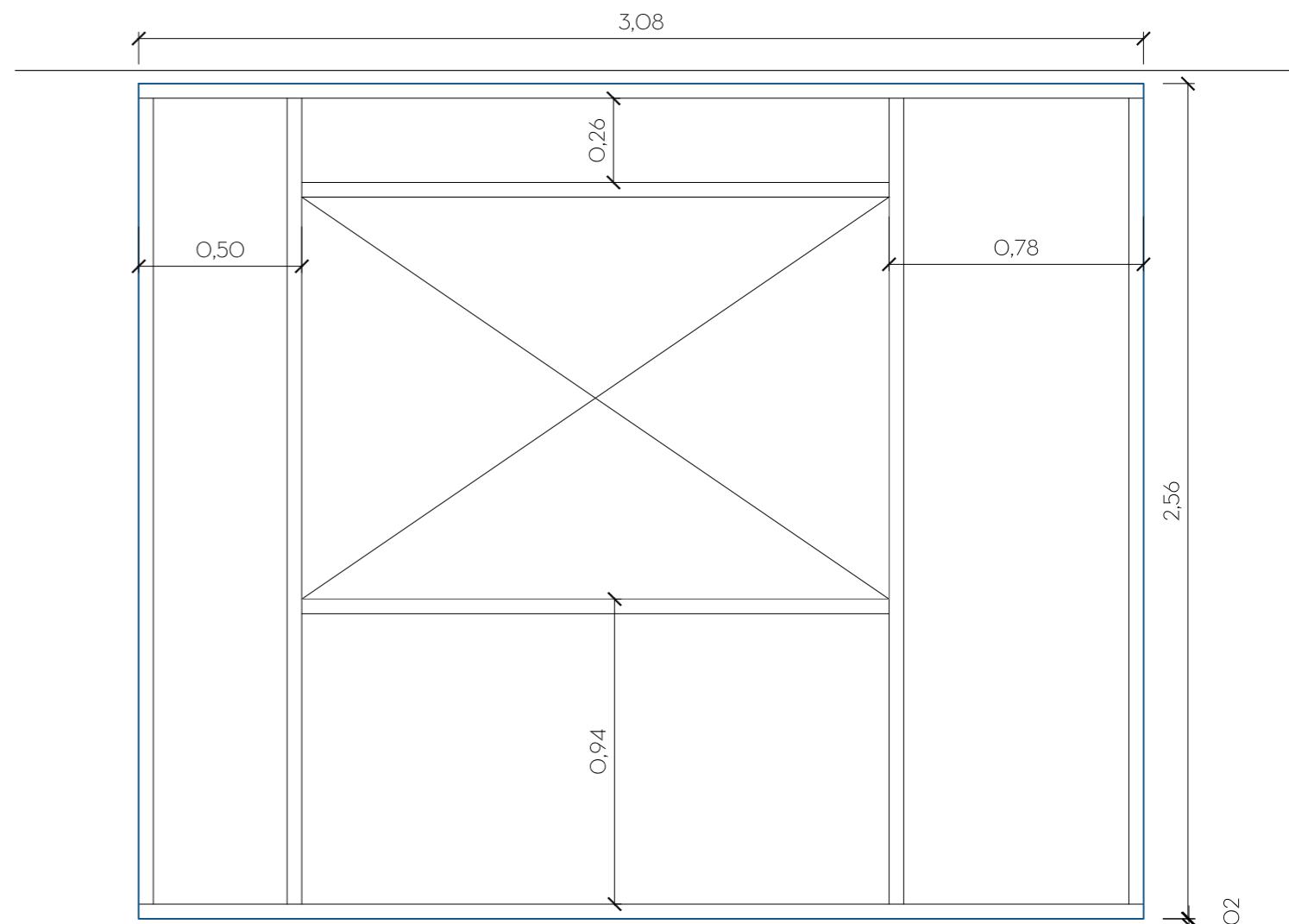
alçat bastidor amb teixit 1:20
