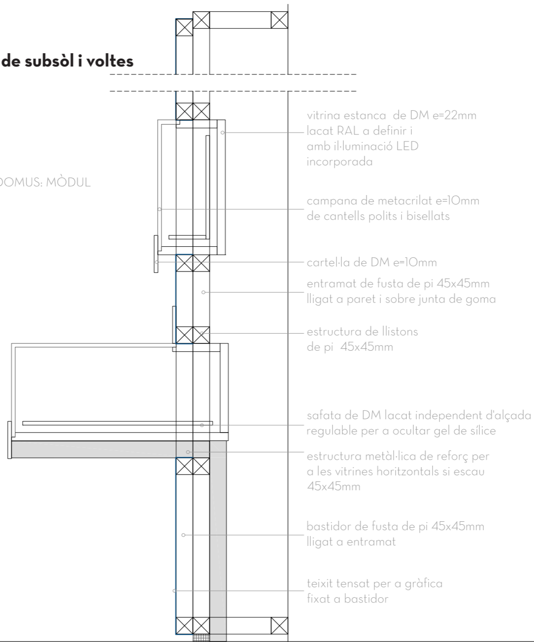
secció 1:10
