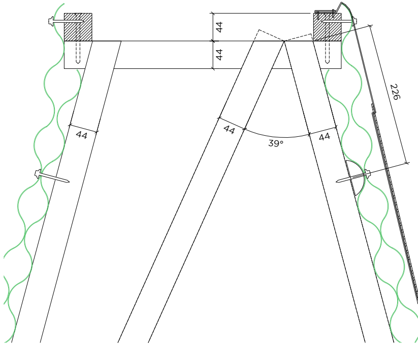
Sección estructura Detalle 2
