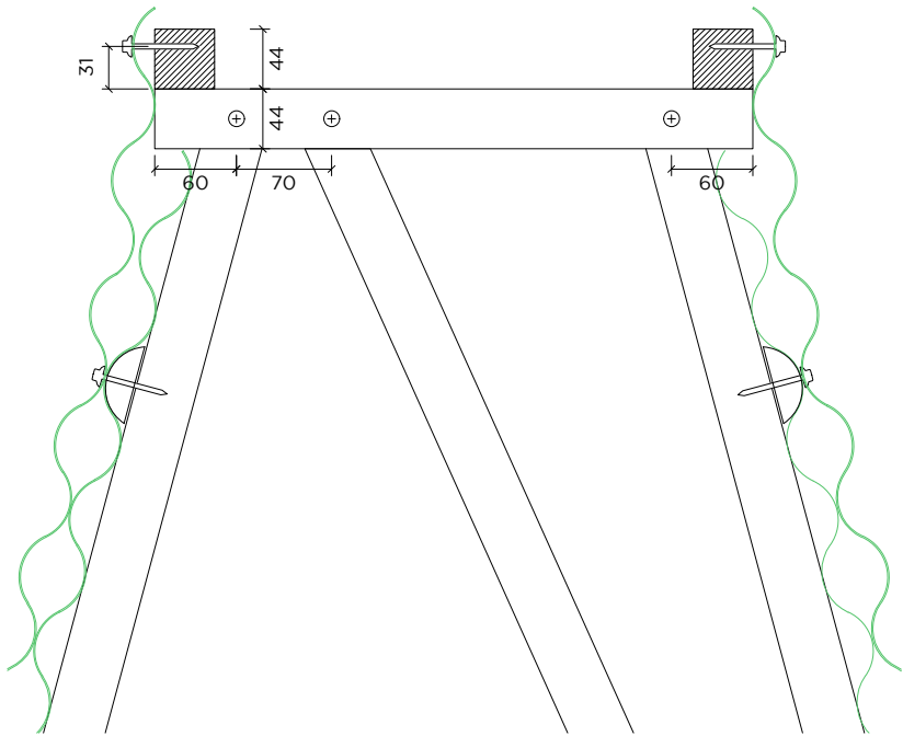
Sección estructura Detalle 1
