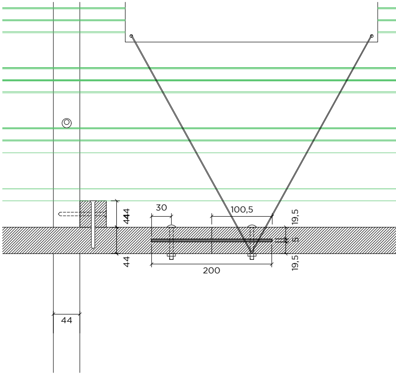
Unión travesaños y fijación placha polistireno Detalle 3
