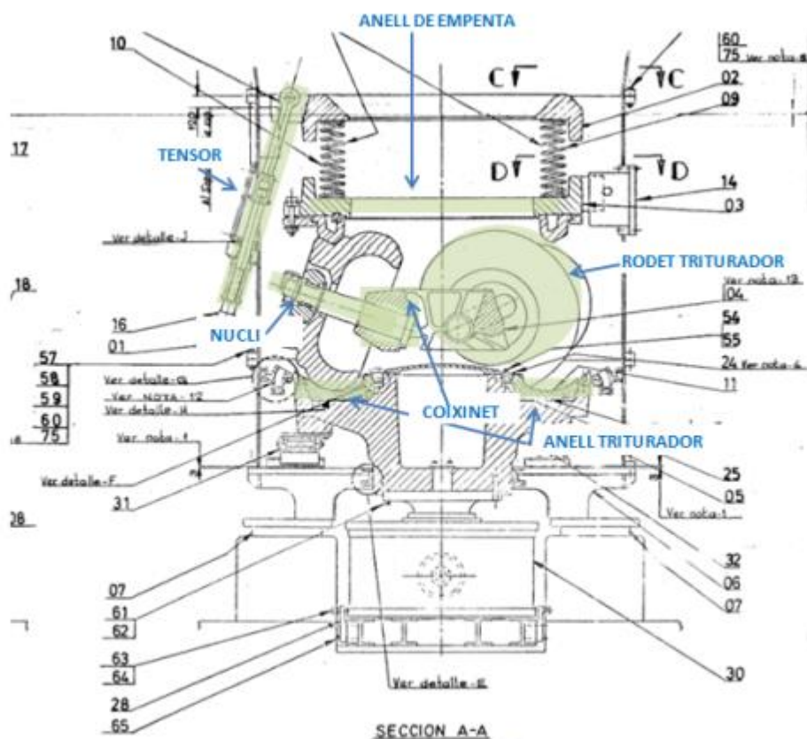
Fragment del plànol de la Maquinista: Conjunto Triturador" seccio A-A.
