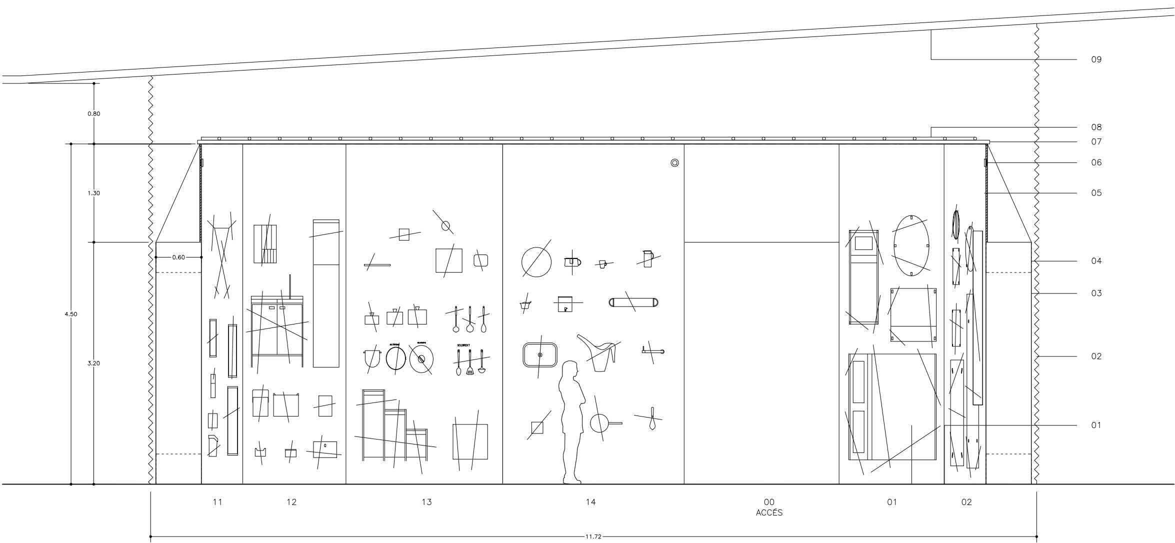
SECCIÓ e:1/50
