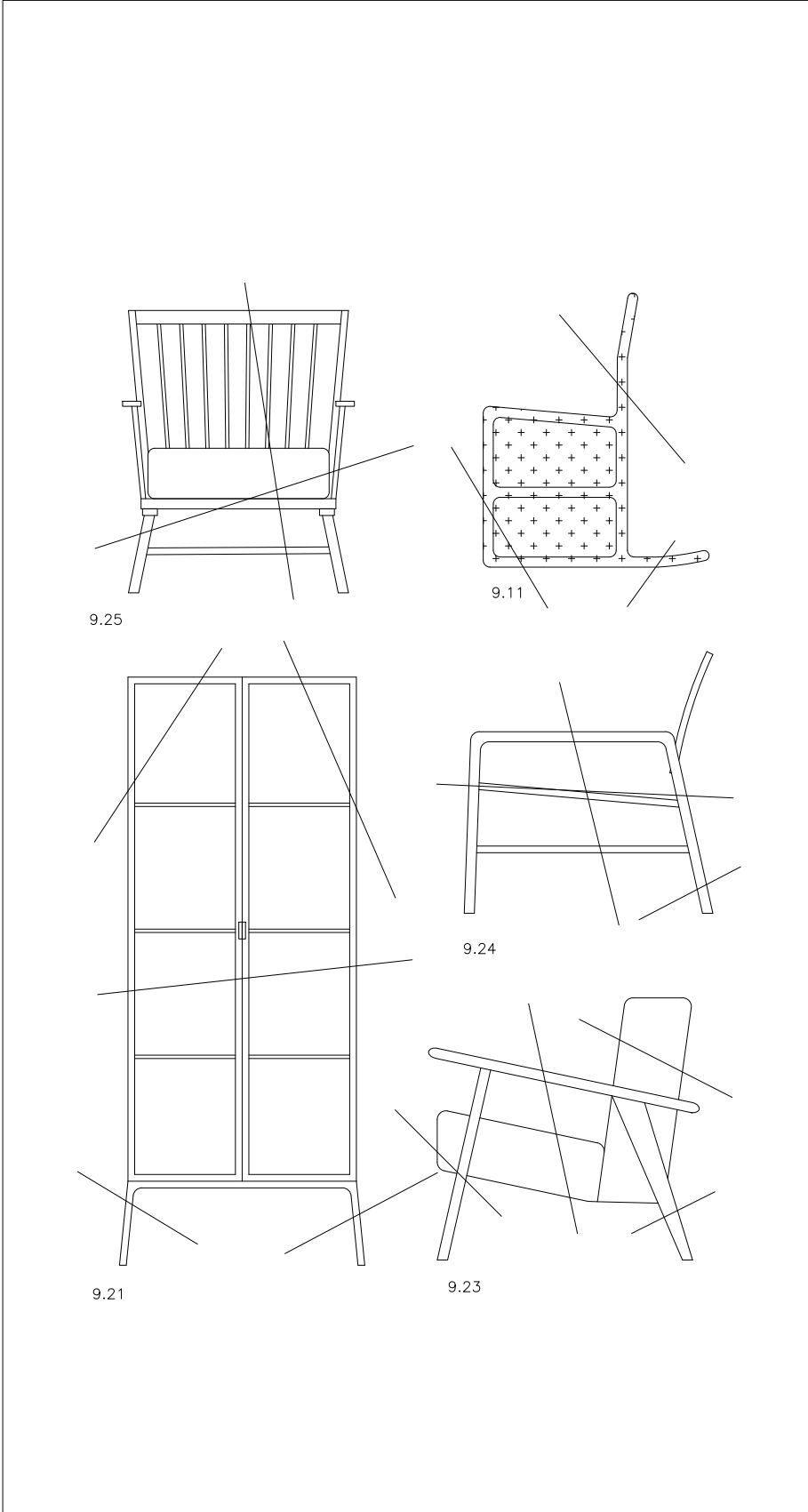
MÒDUL 07 e:1/20
