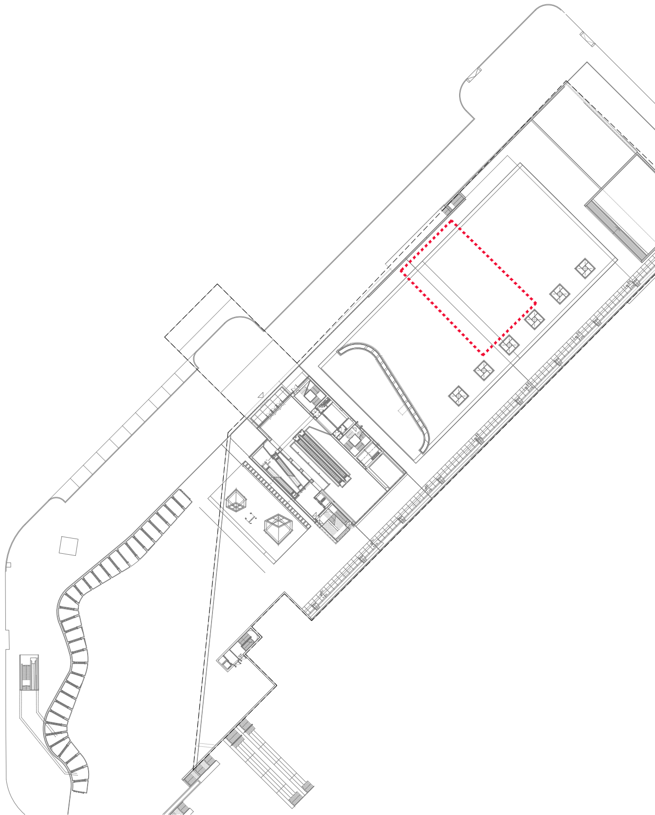
PLANTA SITUACIÓ ESPAI EXPOSITIU e:1/1000
