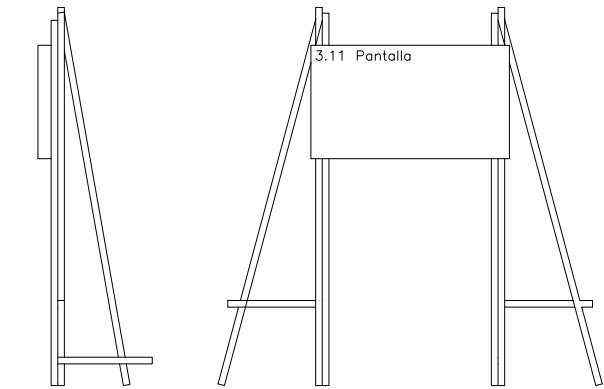
D3.E3 ALÇAT 02
