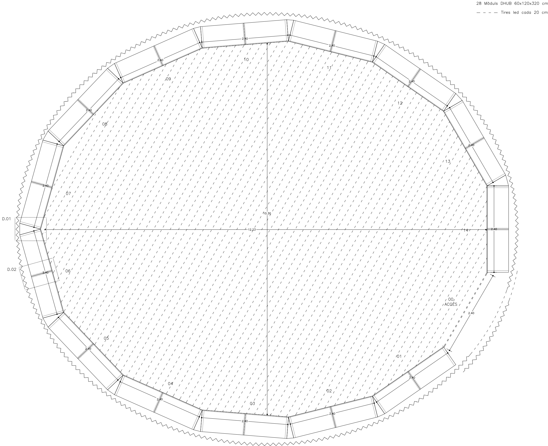
PLANTA e:1/50
