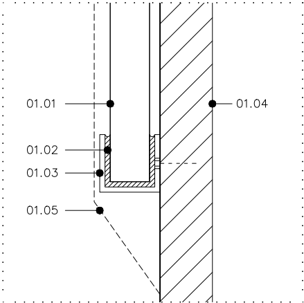
D.01 DETALL DE FIXACIÓ MECÀNICA DE SEGURETAT EXTRA (taules)
