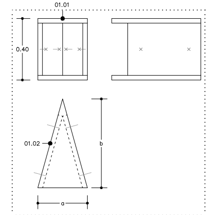
DETALL 01 e:1/25 01.01. Peça triangular superior i inferior en DM de gruix 3cm. Dimensions "a" i "b" variables. 01.02. Peça rectangular en DM de gruix 3cm, cargolada per cara interior a mòduls DHUB.
