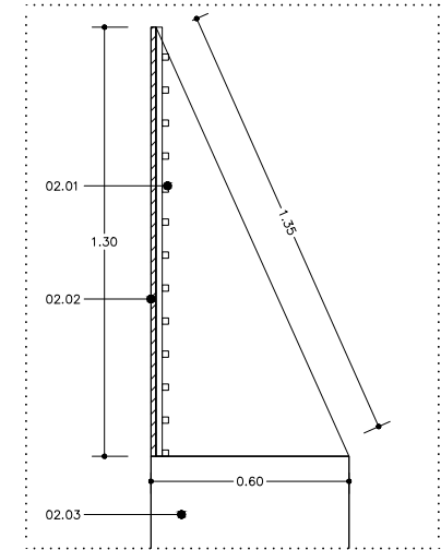
DETALL 02 Secció e:1/25 02.01. Bastidor d'aglomerat de 19mm. 02.02. Suport vertical en DM ignífug de gruix.=15mm 240x130cm acabat a definir. 02.03. Mòduls DHUB 60x120x320 cm.
