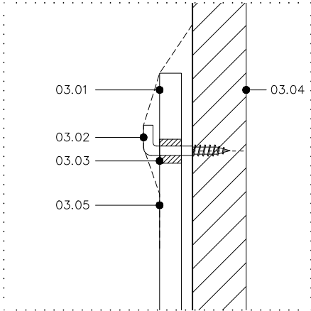
D.03 DETALL DE FIXACIÓ MECÀNICA DE SEGURETAT EXTRA (peçes petites)
