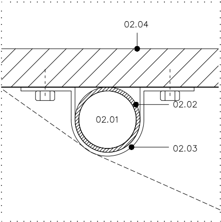
D.02 DETALL DE FIXACIÓ MECÀNICA DE SEGURETAT EXTRA (cadires)
