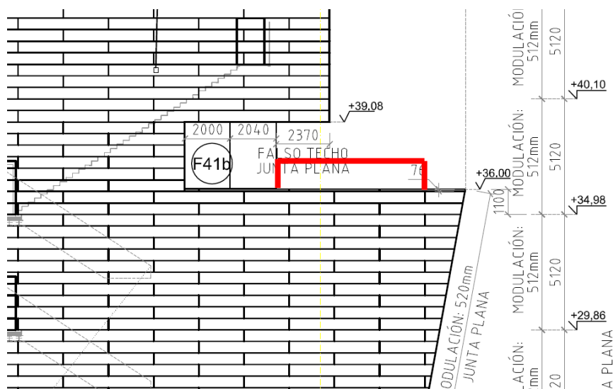
Plànol alçat ubicació vidre.
