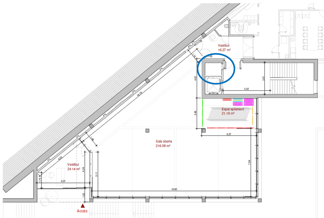
Planta primera CUB
