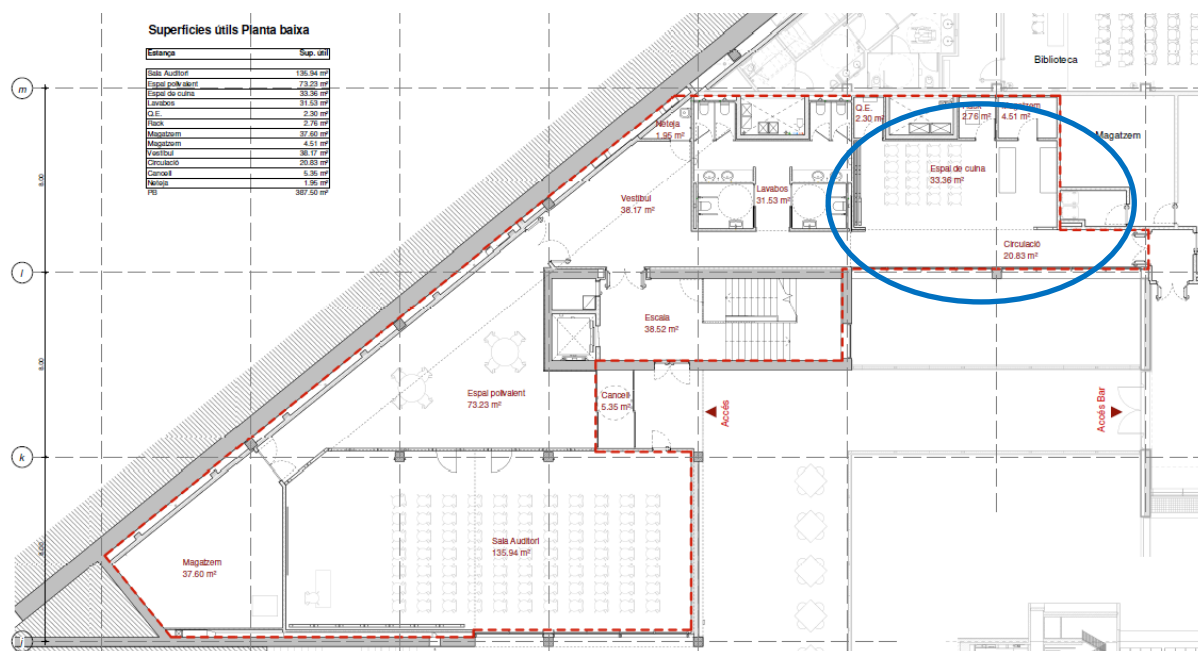
Planta baixa CUB. Zona actuació.
