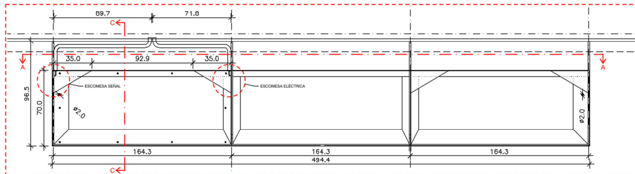
PLANTA - ESTRUCTURA E:1/20
