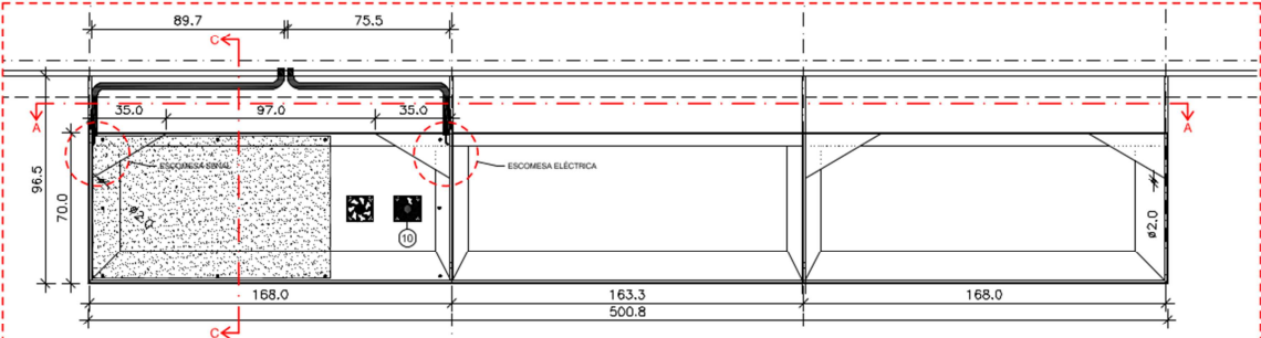
PLANTA - ESTRUCTURA E:1/20
