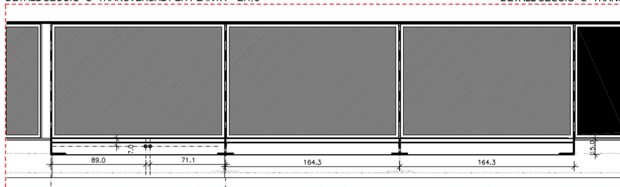
SECCIÓ POSTERIOR A E:1/20
