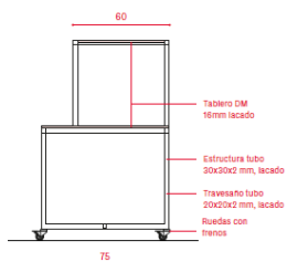
Sección, esc. 1:20
