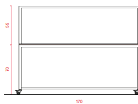
Alzado, esc. 1:20
