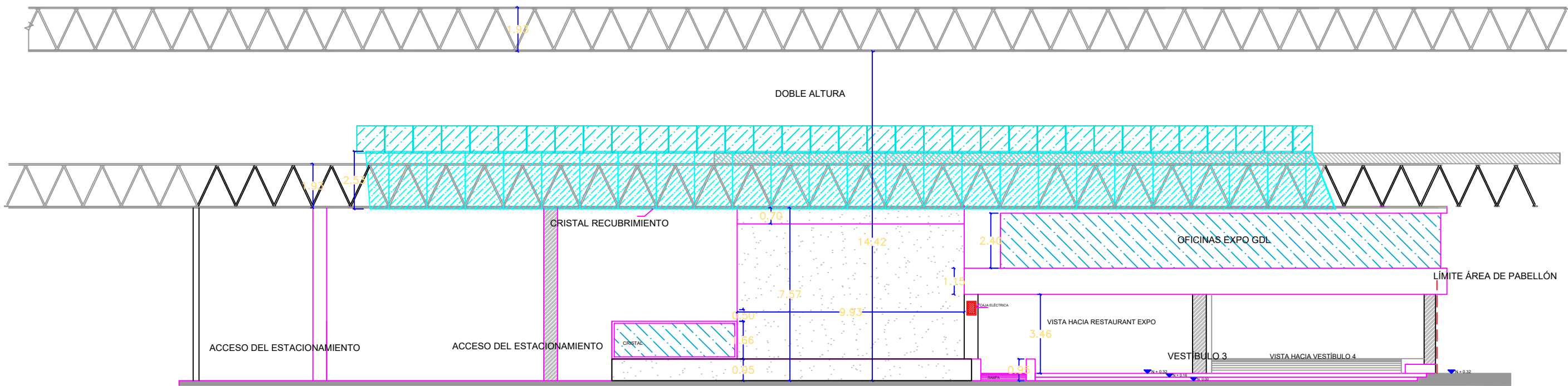
ALZADO B VISTA HACIA VESTÍBULO 3
