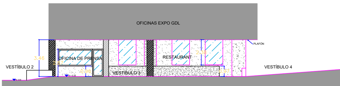
ALZADO D VESTÍBULO 3
