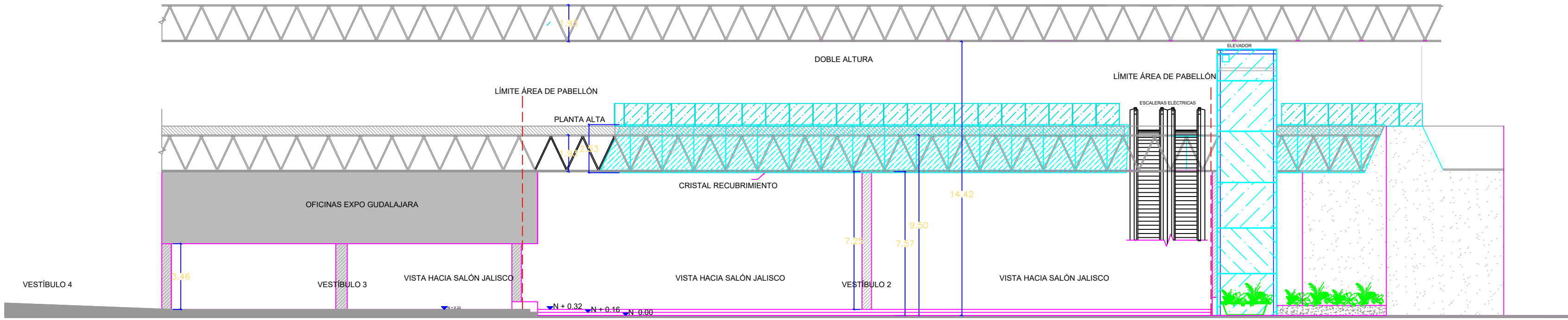
ALZADO A VISTA HACIA SALÓN JALISCO
