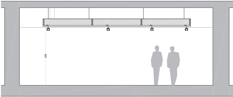
SECCIÓ TRANSVERSAL. S3 E.1:100
