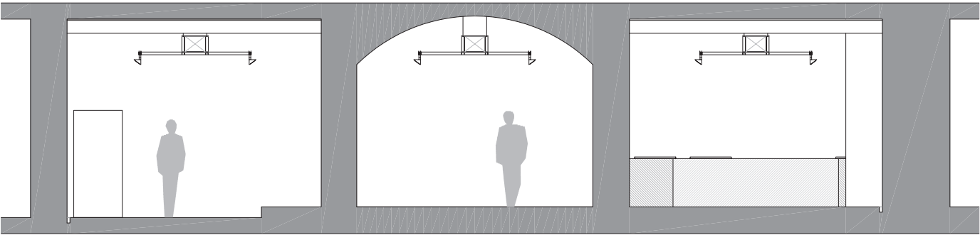
SECCIÓ LONGITUDINAL.S1 E.1:100
