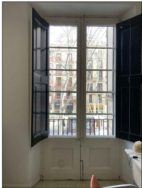
ESTAT ACTUAL AMB VIDRE SIMPLE. DETALLS 1 I 2
