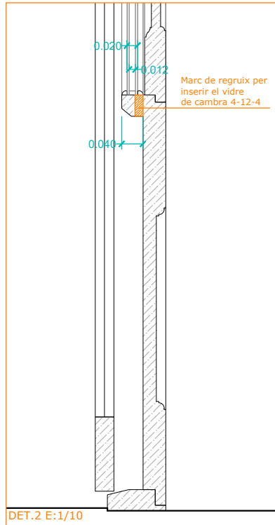
PROPOSTA OPCIÓ 2. REHABILITACIÓ AMB VIDRE DE CAMBRA, DOBLE VIDRE. DETALLS 1 I 2
