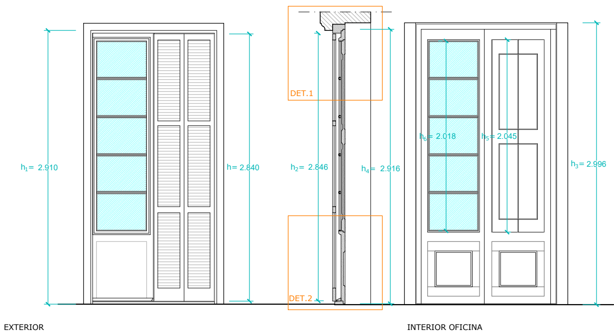
ALÇAT EXTERIOR E: 1/40
