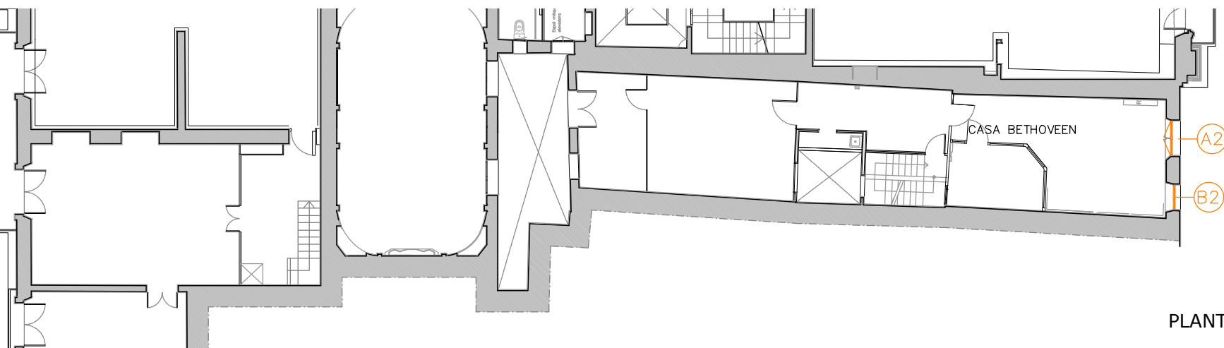
PLANTA TERCERA
