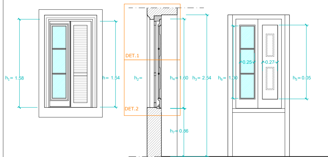
ALÇAT EXTERIOR E: 1/40
