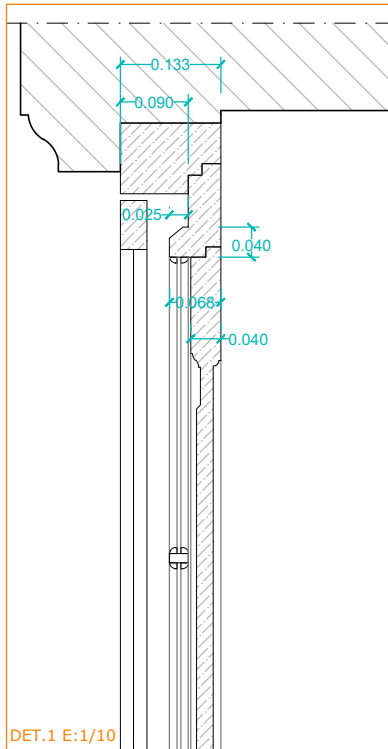
ESTAT ACTUAL AMB VIDRE SIMPLE. DETALLS 1 I 2
