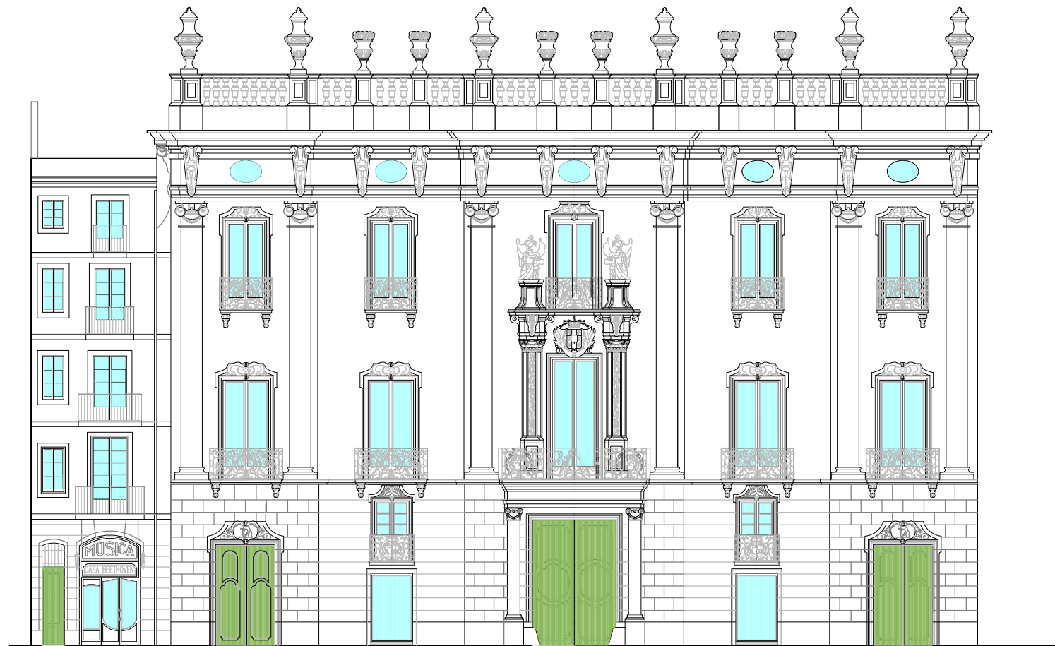
ALÇAT EDIFICI VIRREINA I CASA BEETHOVEN, FAÇANA PRINCIPAL A LA RAMBLA E: 1/200
