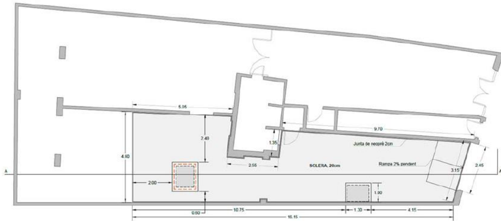
Secció actual paviment de planta baixa
