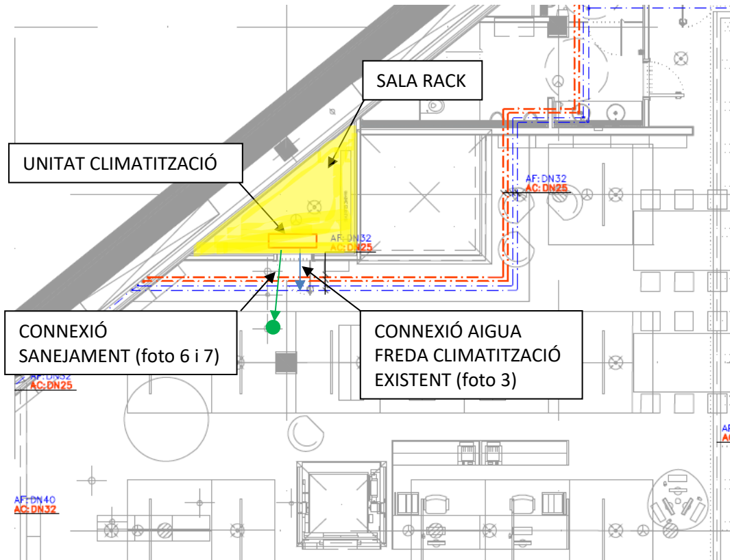
PLÀNOL UBICACIÓ SALA RACK PLANTA PRIMERA
