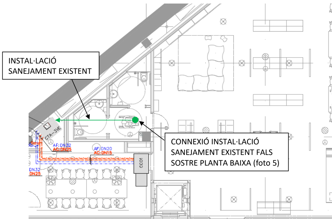
PLÀNOL UBICACIÓ CONNEXIÓ SANEJAMENT PLANTA BAIXA
