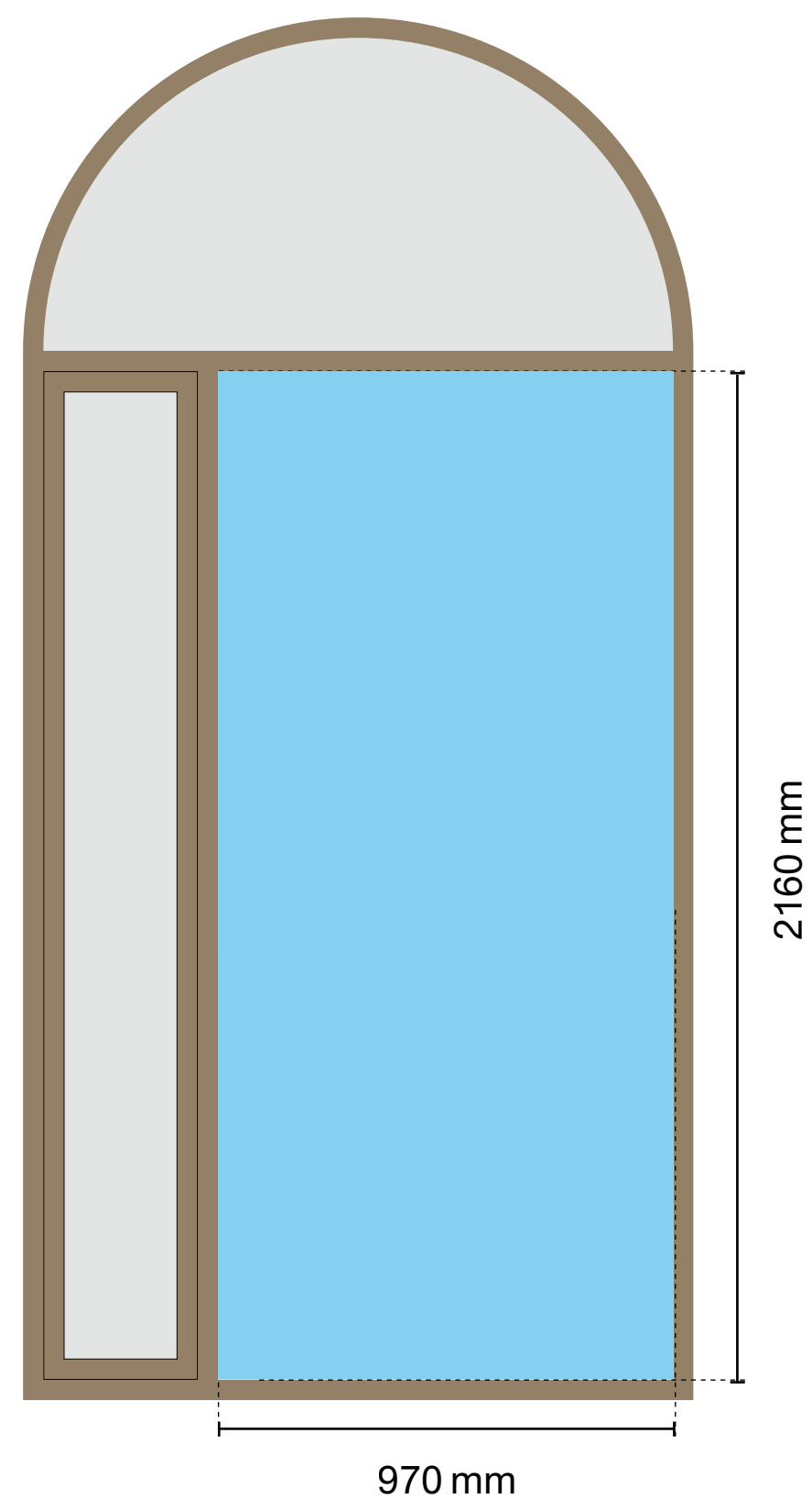
2.1.1. Vinil a l'àcid per finestra model A
