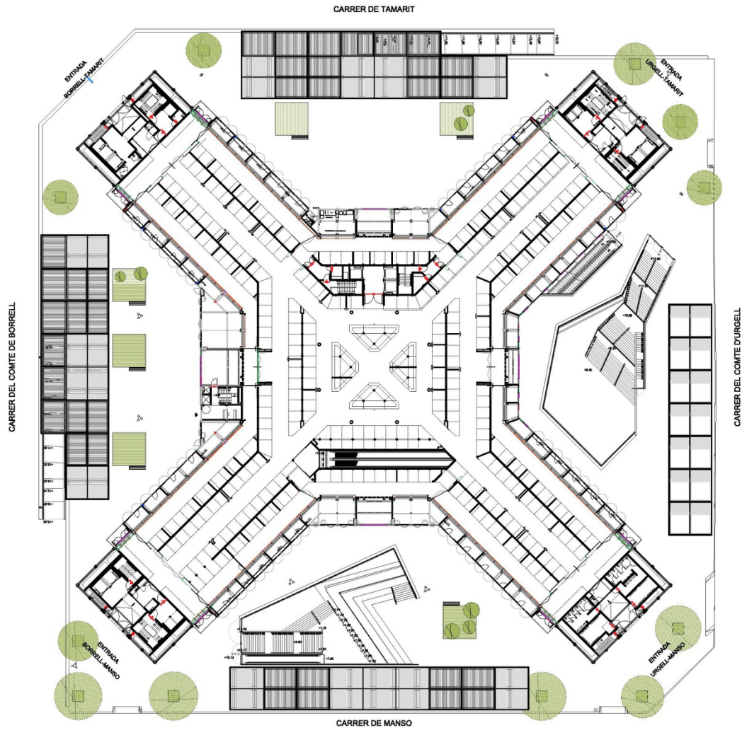
Planta baixa Mercat de Sant Antoni
