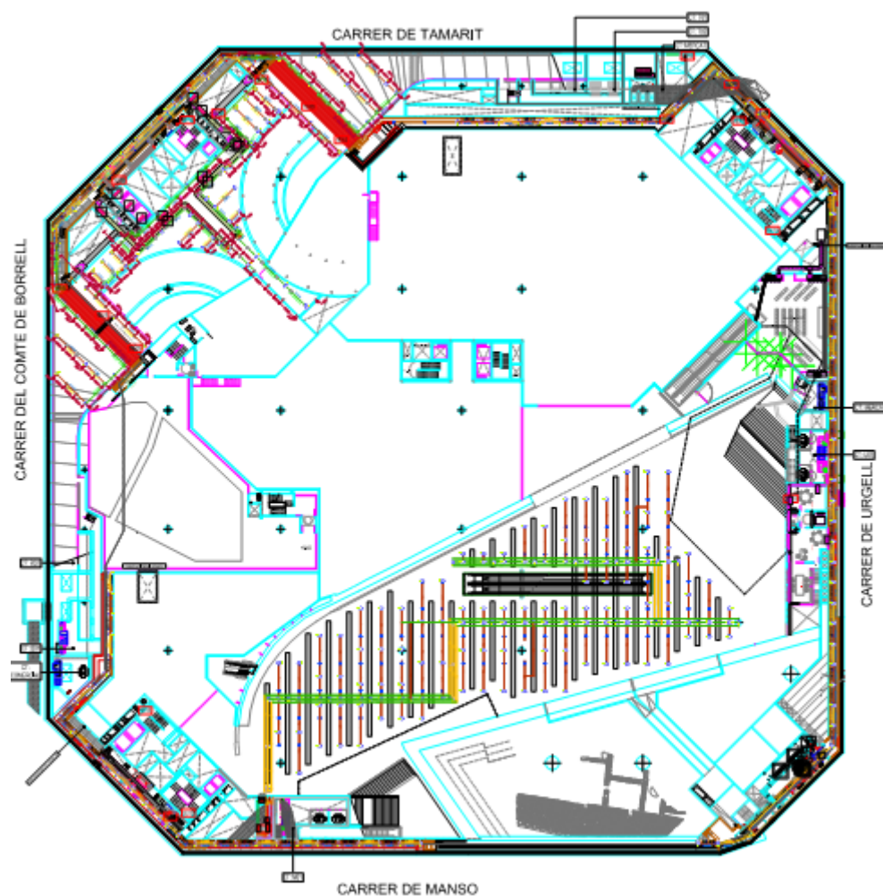
Planta soterrani 1 Mercat de Sant Antoni (fossat)
