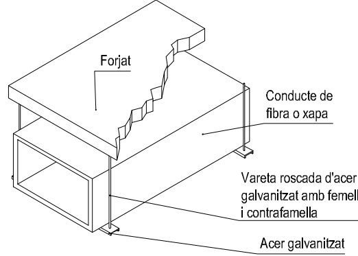
Detall subjecció de conductes
