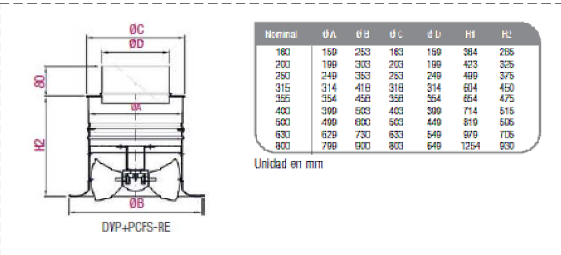
Detall difusor d'impulsió
