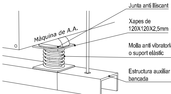
Detall molla antivibratòria
