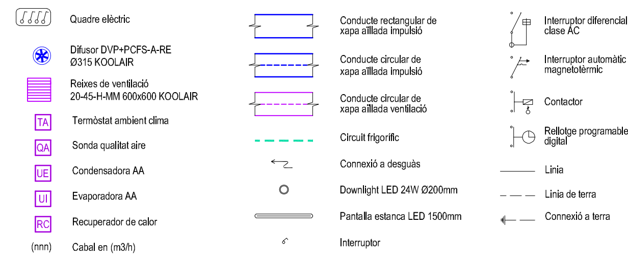
Simbologia
