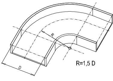
Detall radi típic
