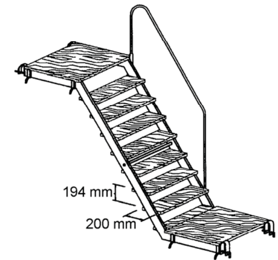
DETALL D'UN TRAM
