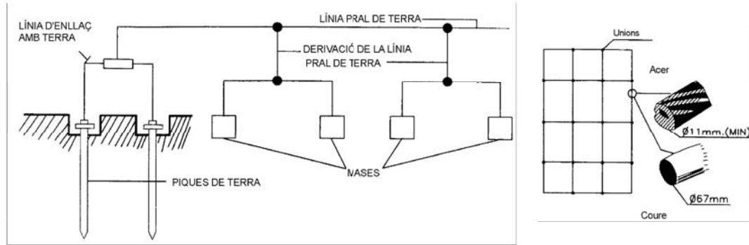
ESQUEMA D'UN CIRCUIT DE POSTA A TERRA
