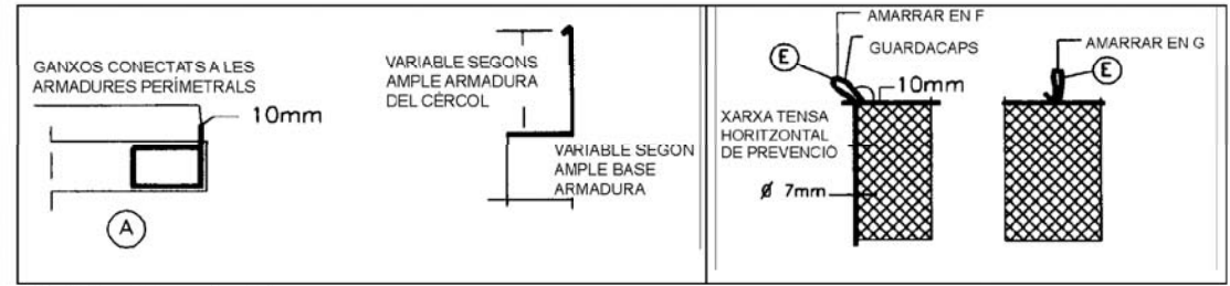
DETALL DE GANXO
