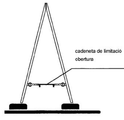
ESCALA DE TISORA
