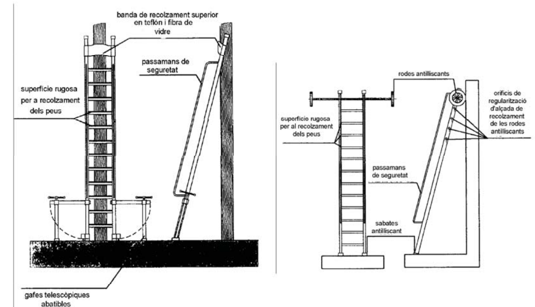
ESCALA ANTIVOLCATGE PER A ACCÈS A ELEMENTS ESTRETS
