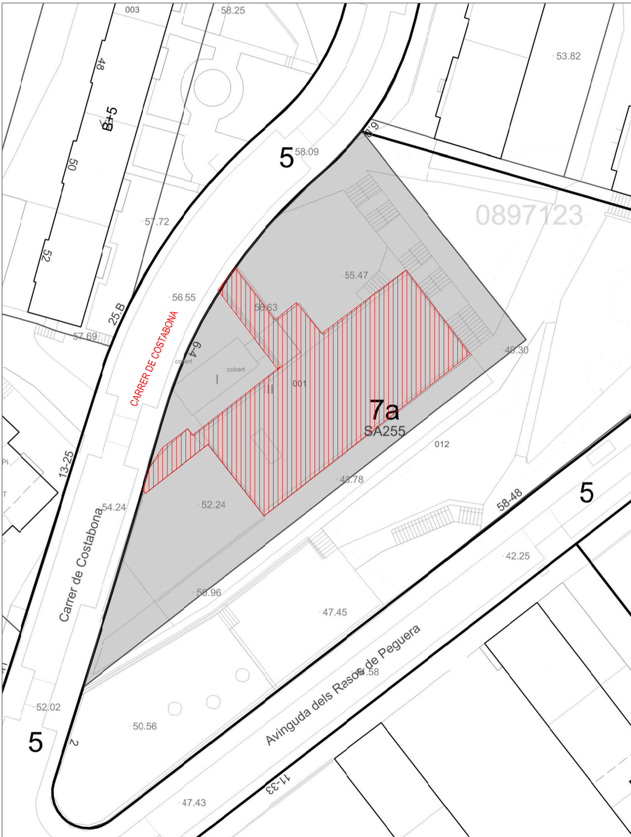
Emplaçament E.1:500
